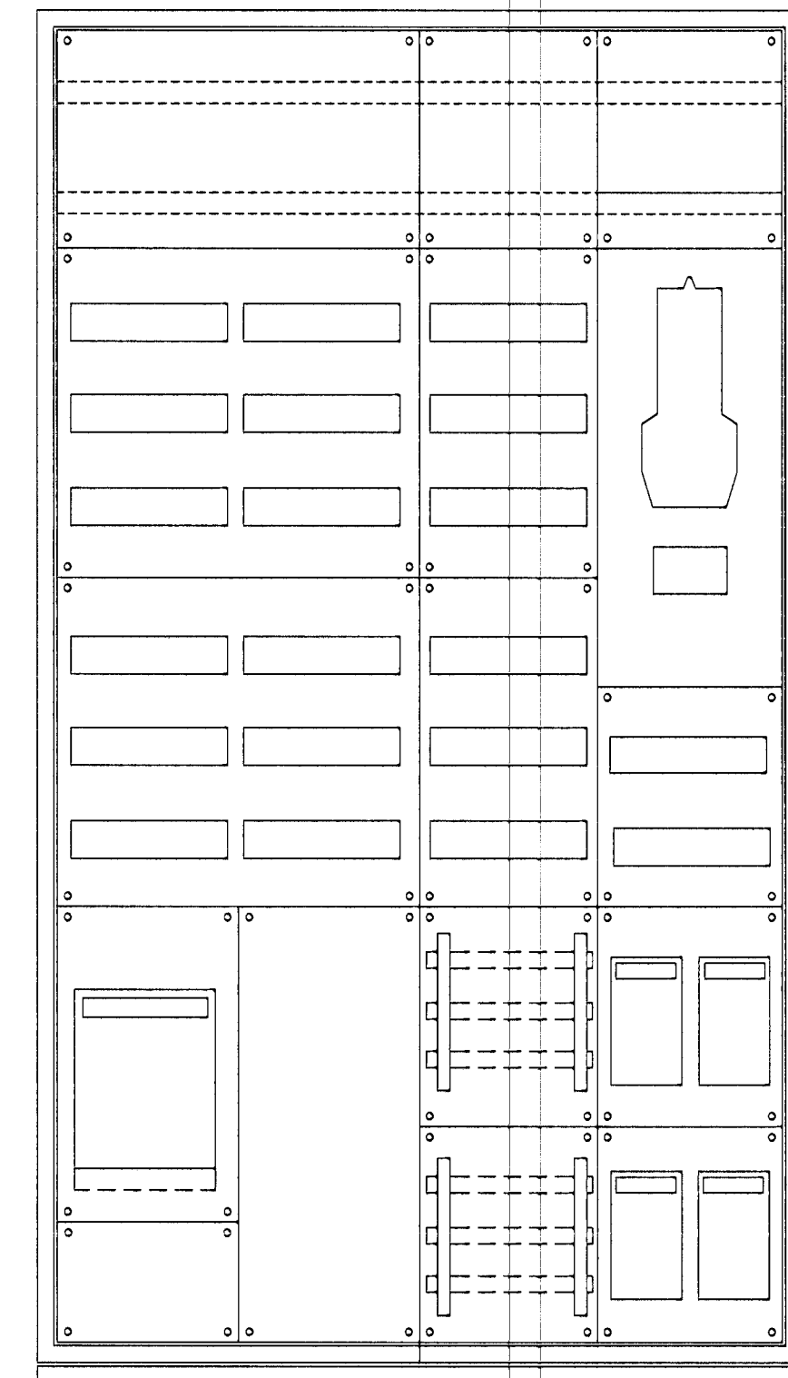
Útlit að aðaltöflu mkv. 1:20
