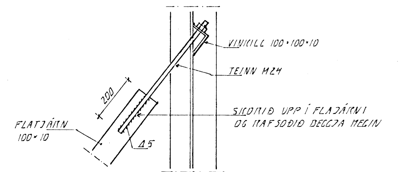
VINDSTÍFING DEILI 1, 1:10
