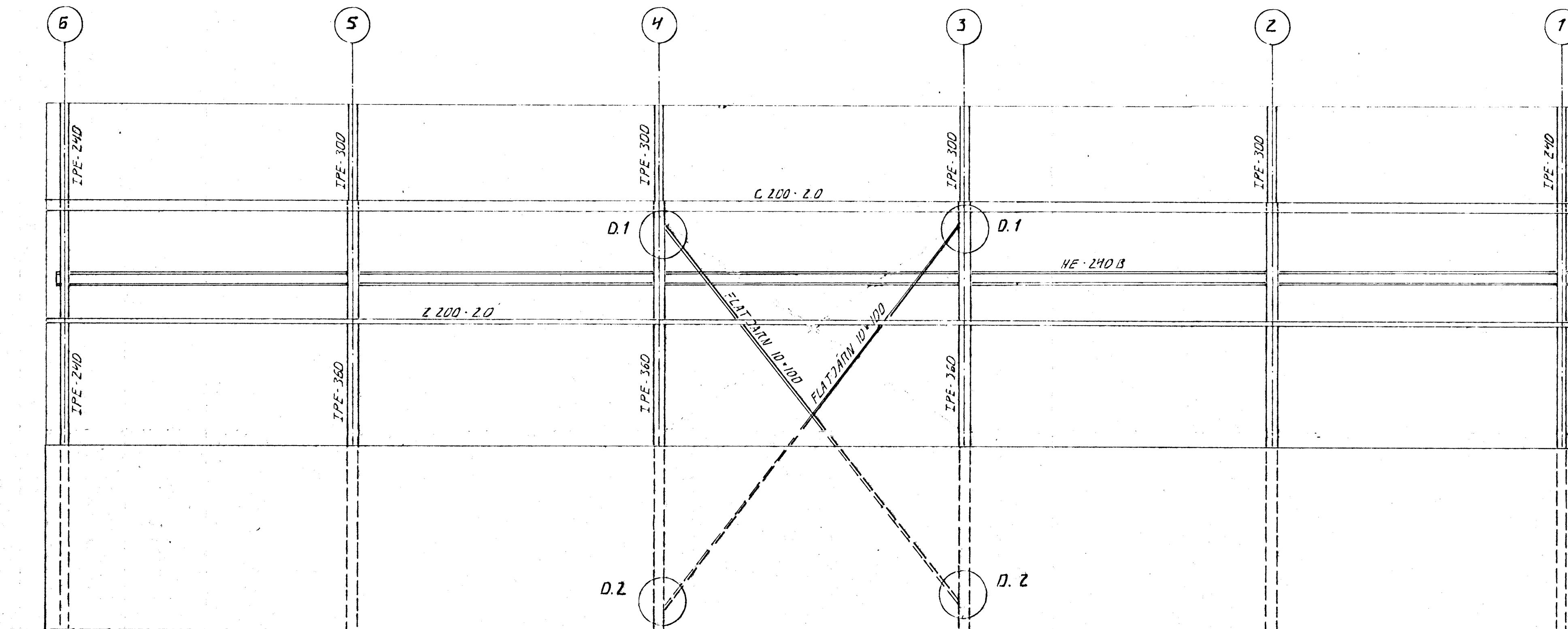
ÁSYND SUB-AUSTUR, 1:50
