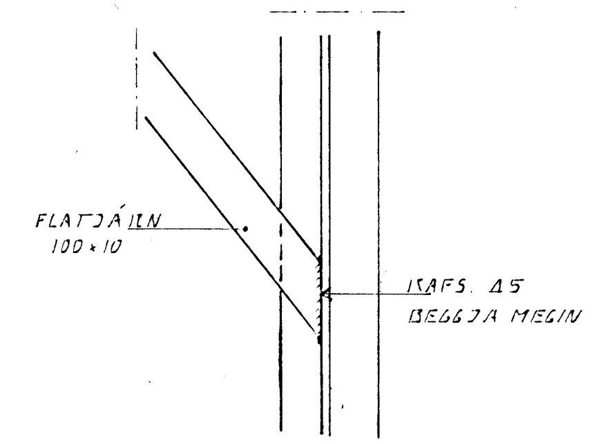
VINDSTÍFING DEILI 2, 1:10
