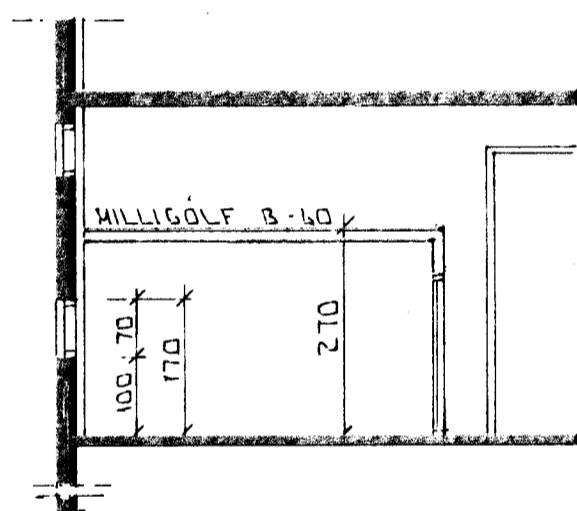
SNID B-B 1:100
