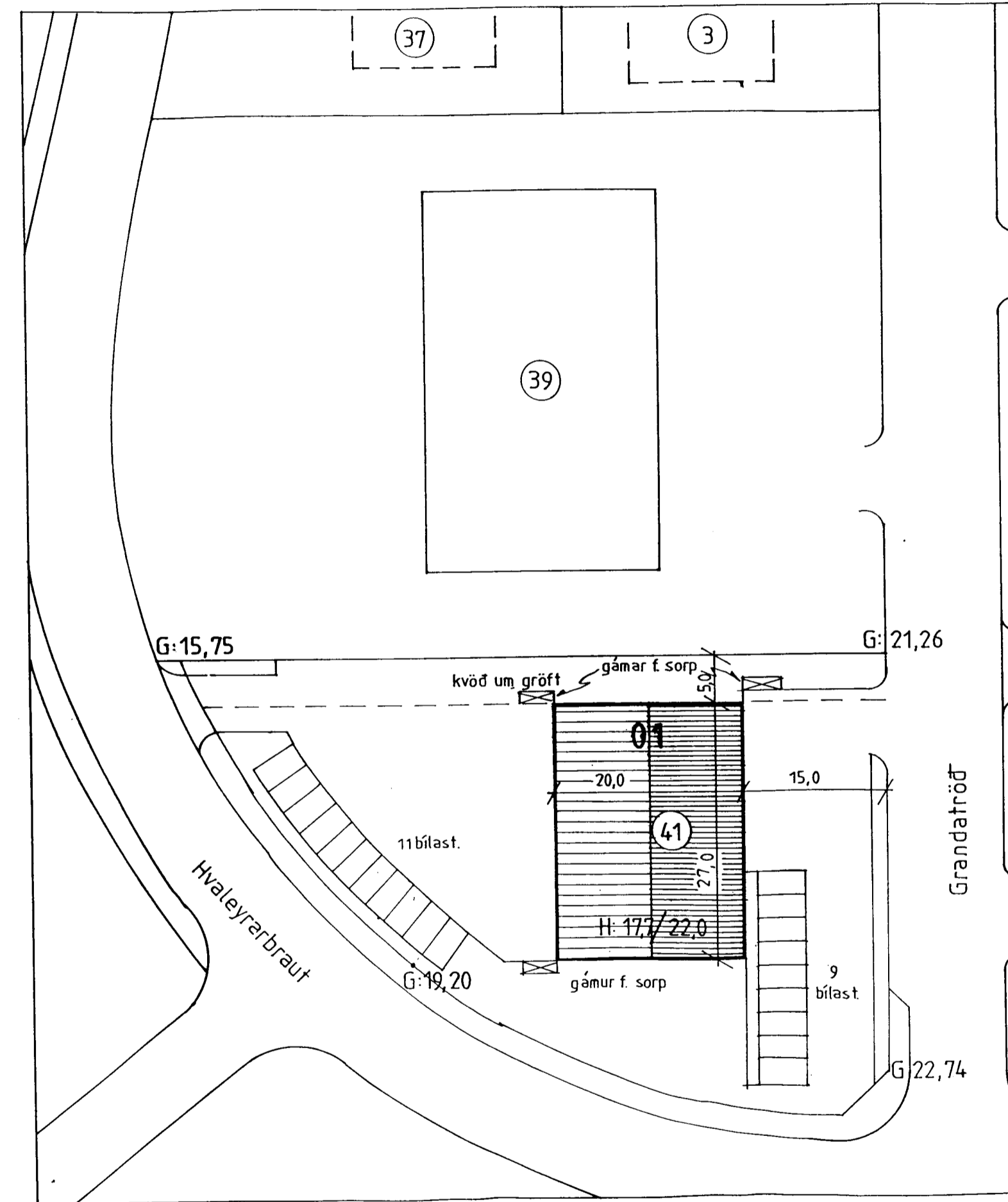
afstöðumynd 1:500
