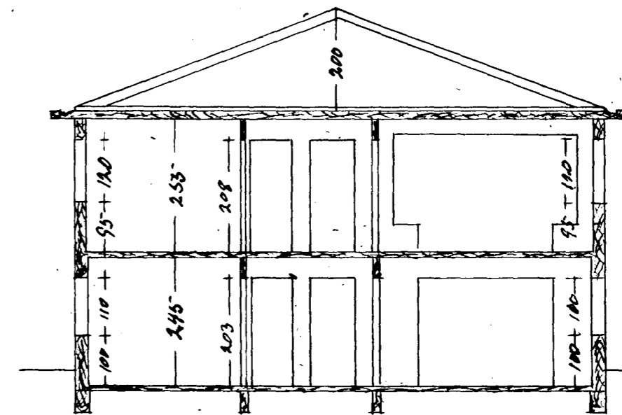
Þverskurður
