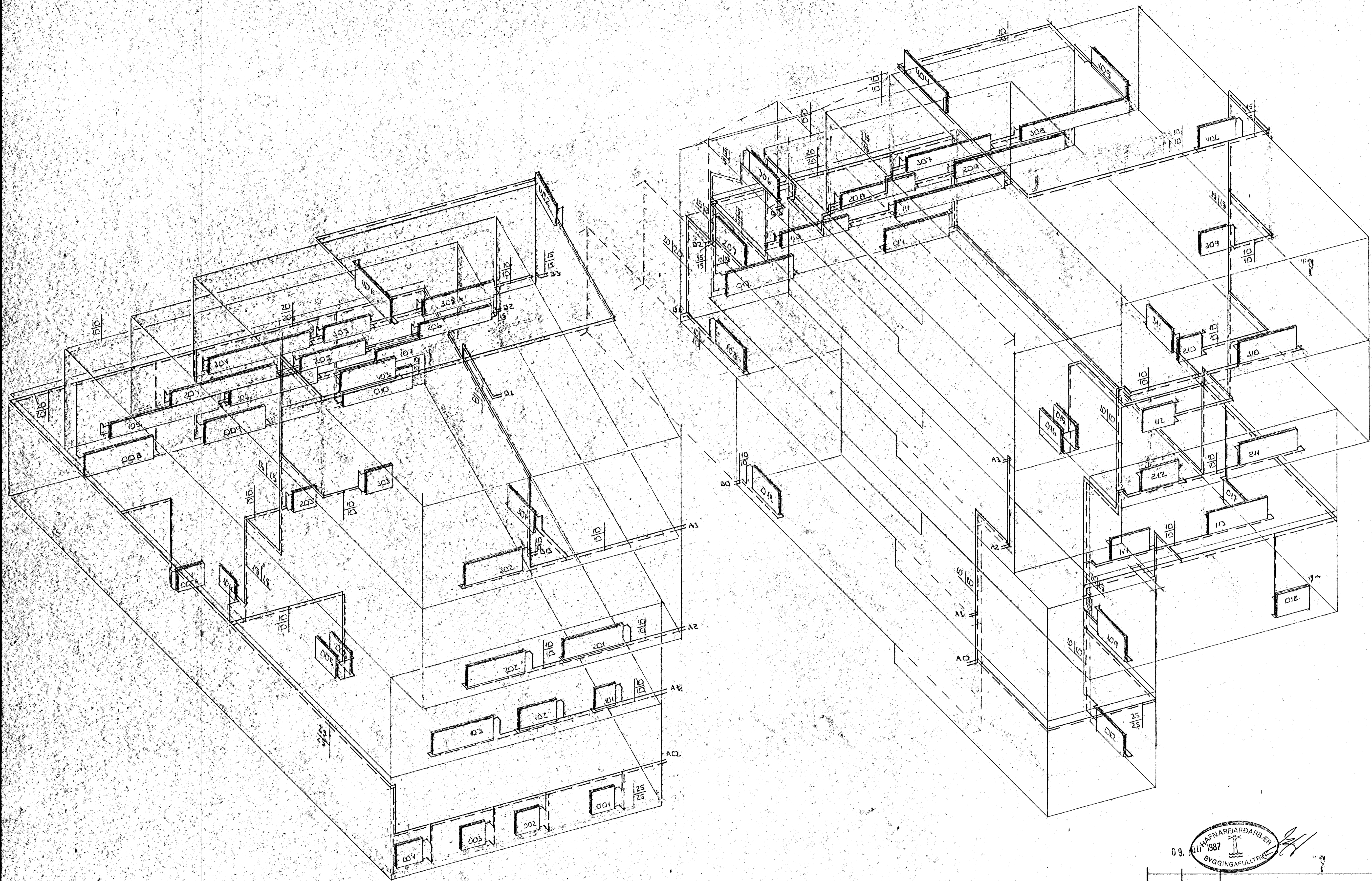
RÚMMYND HITALAGNA 1:50
