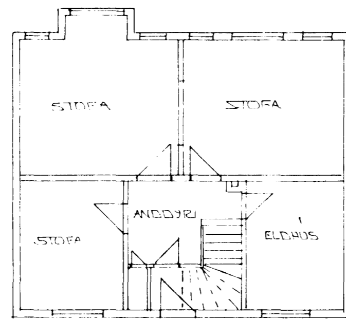
I. HÆÐ - 1:100
