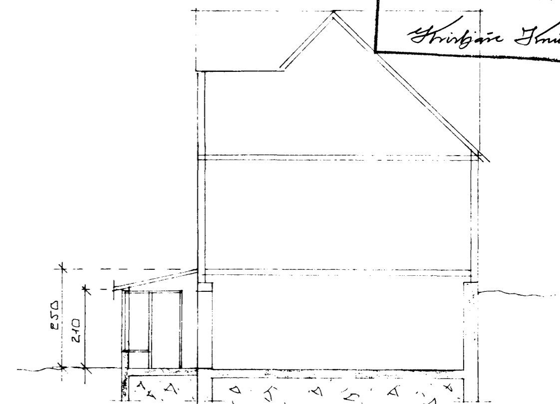
SKURÐUR A-A - 1:100
