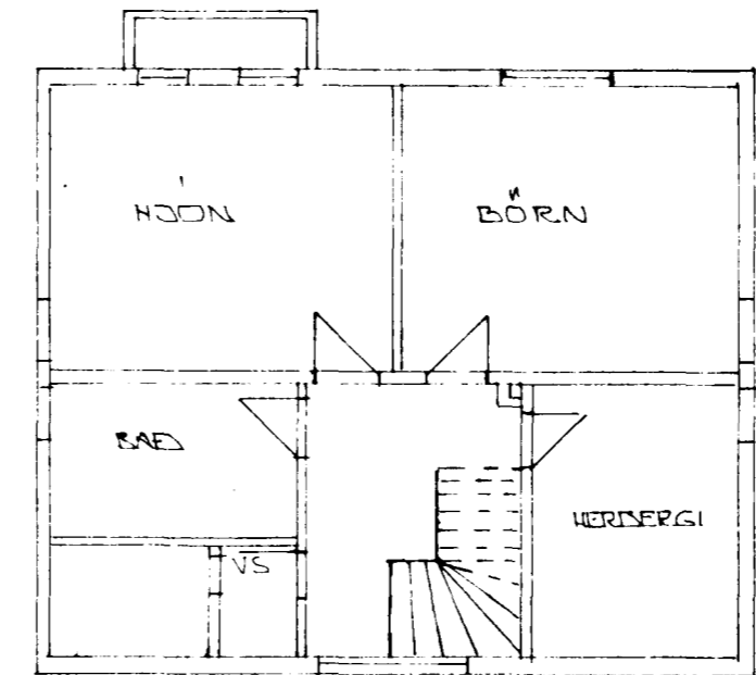
II. HÆÐ - 1:100
