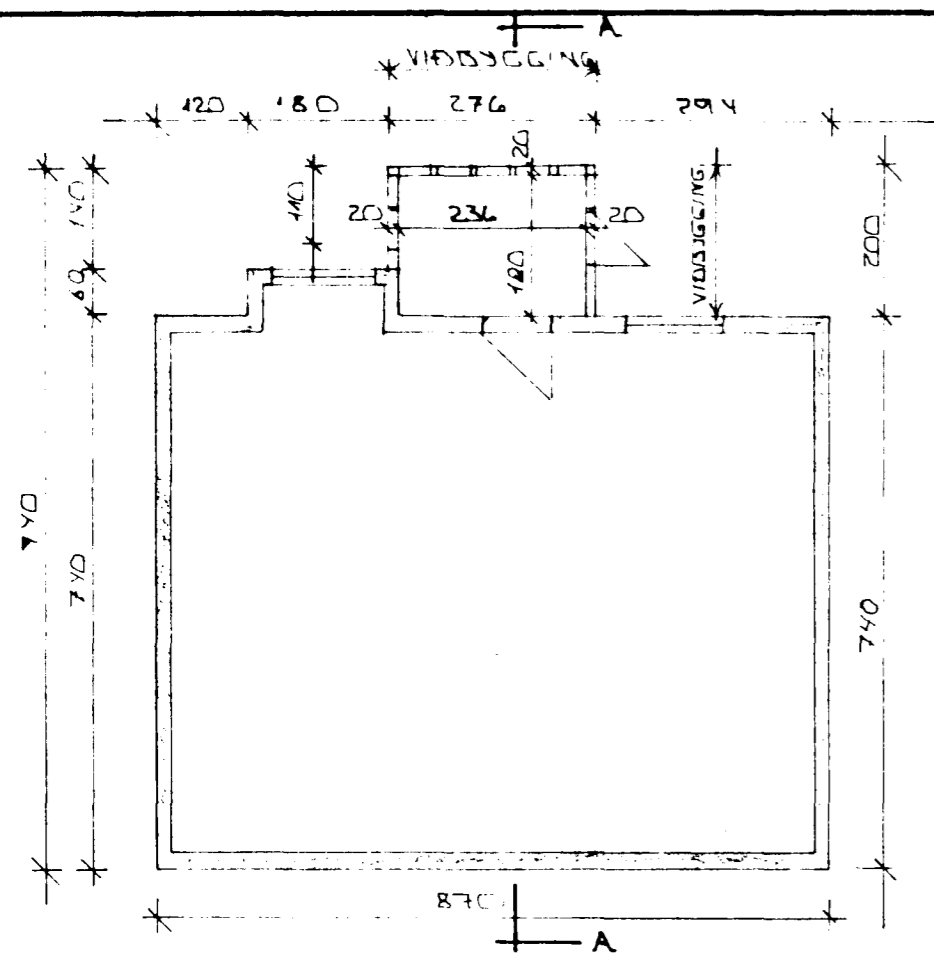
KJALLARI - 1:100
