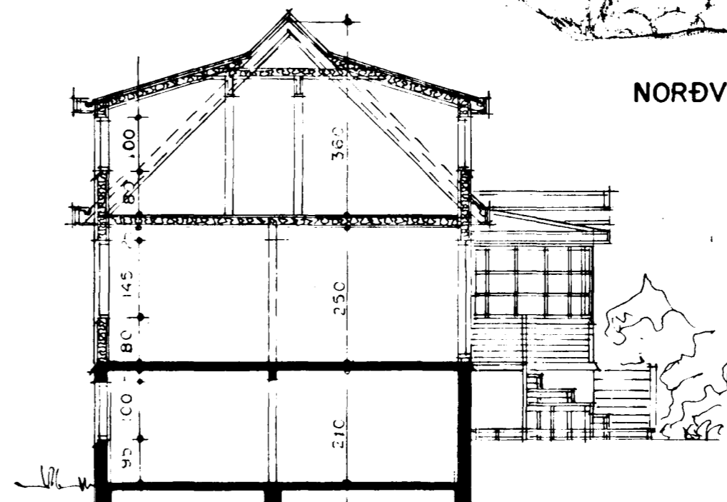
SNEIÐING A-A
