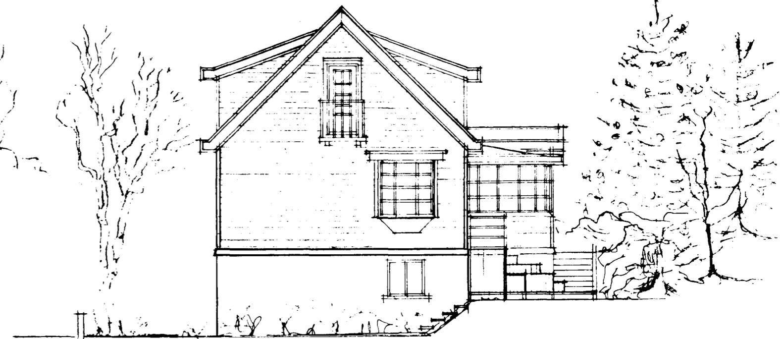
SUÐAUSTURHLIÐ
