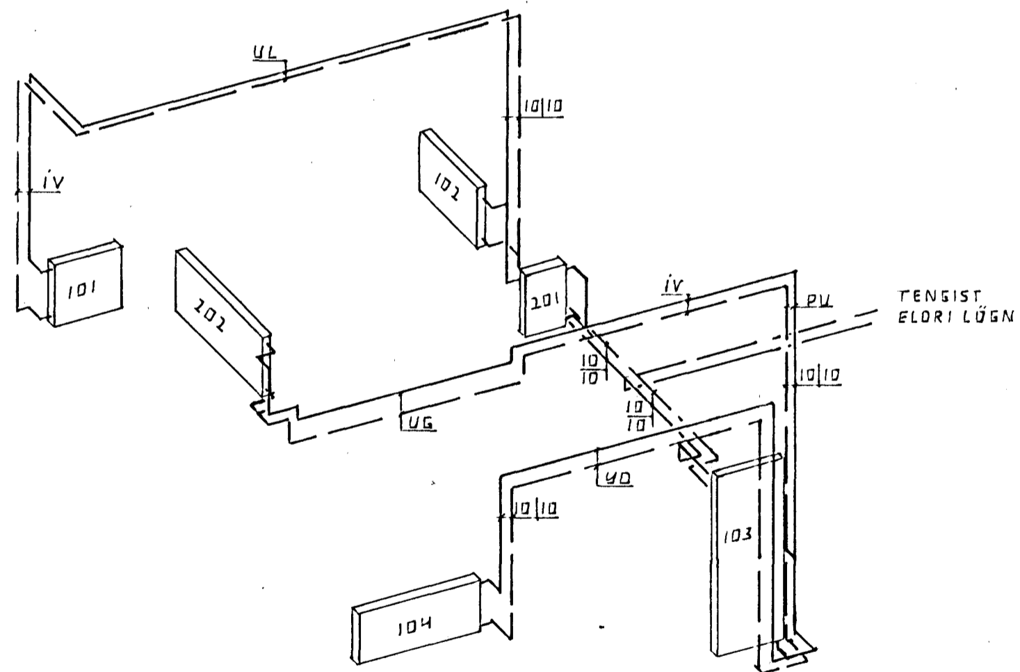
RÚMMYND HITALAGNA 1:50
