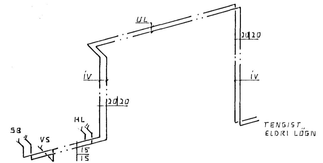
RÚMMYND VATNSLAGNA 1:50
