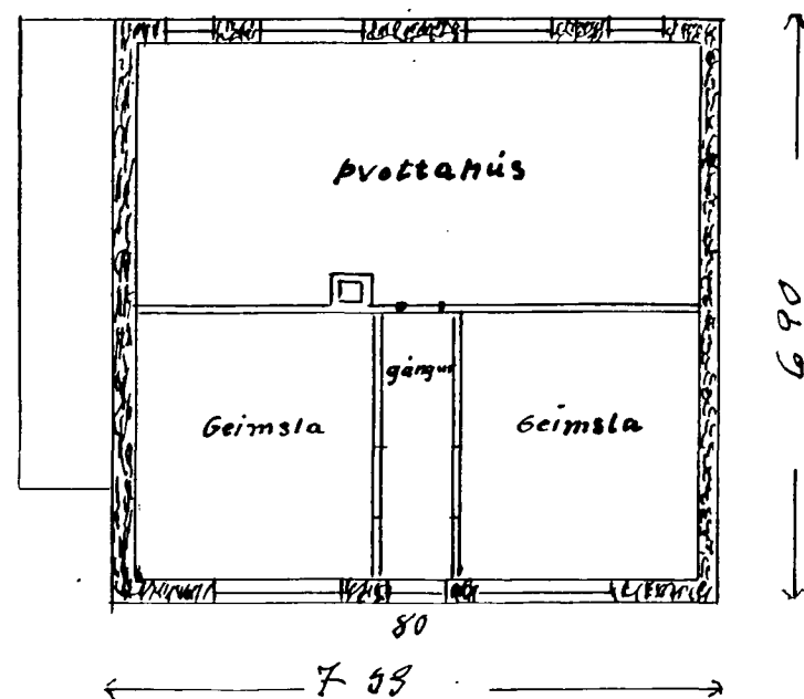
Kjallari.
