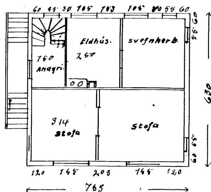
1. hæð.
