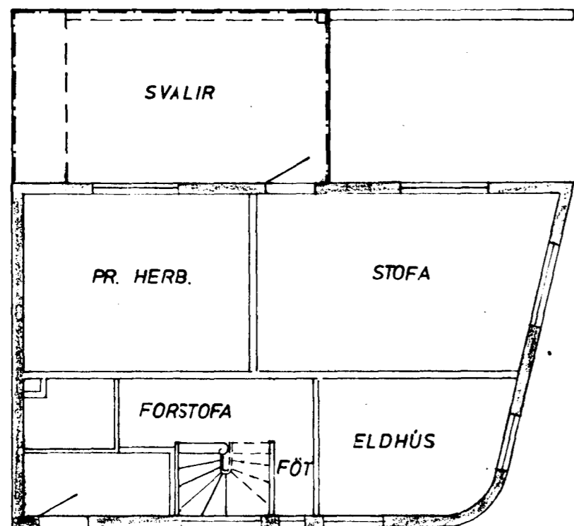
GRUNNMYND HÆÐAR 1:100
