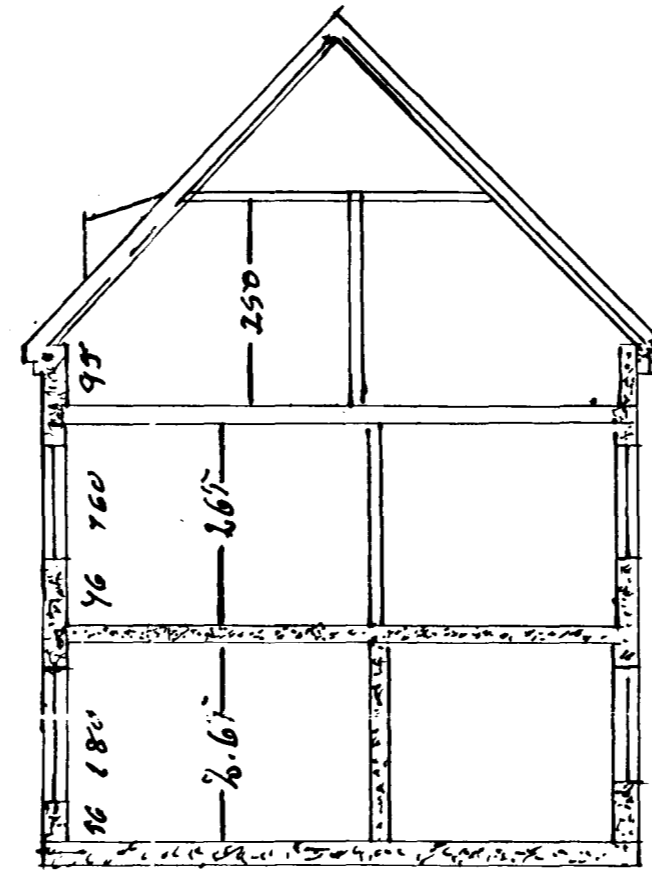
ÞVEASKURÐUR A-A
