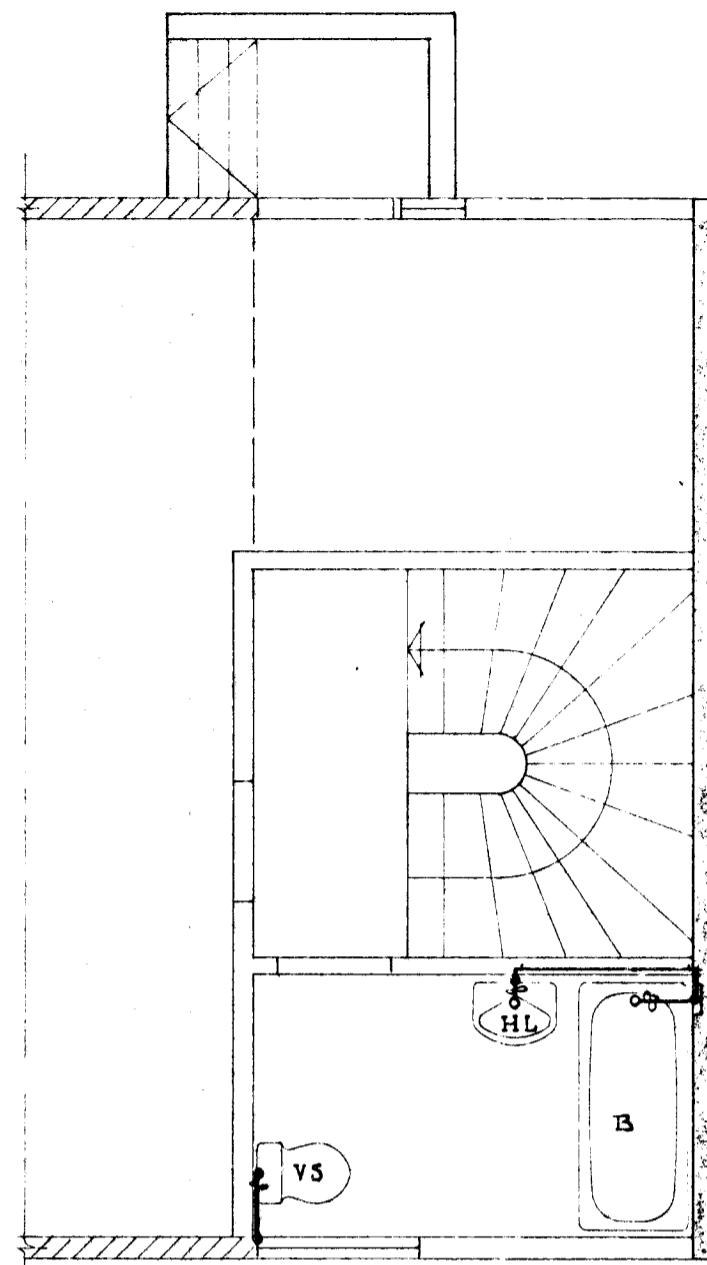
1. HÆÐ 1:50
