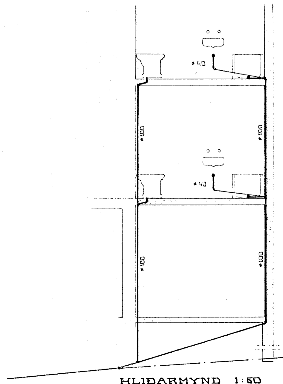
HLIÐARMYND 1:50
