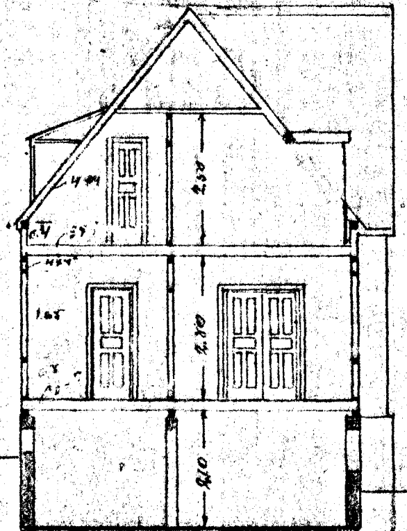
SKURÐUR A-A
