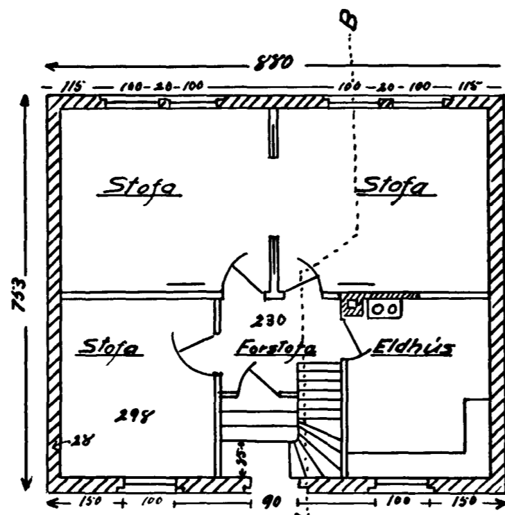
Stofuhæð
