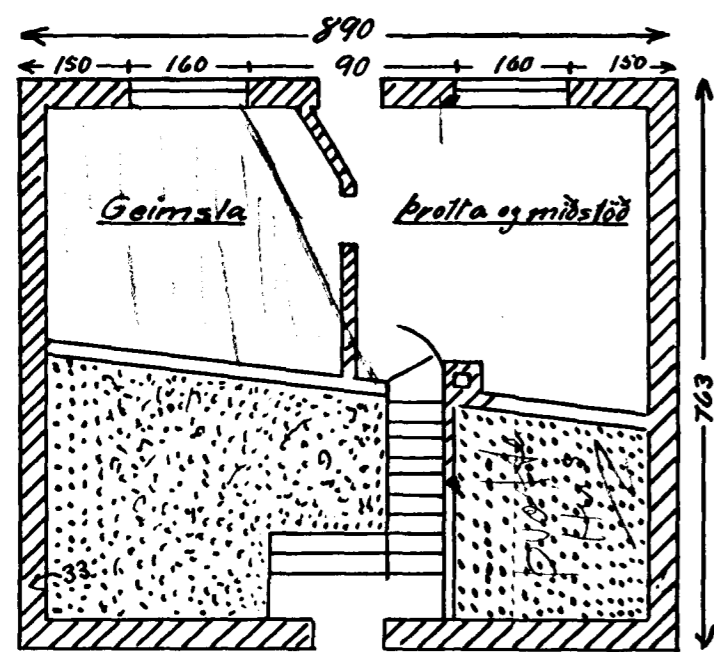
Kjallari
