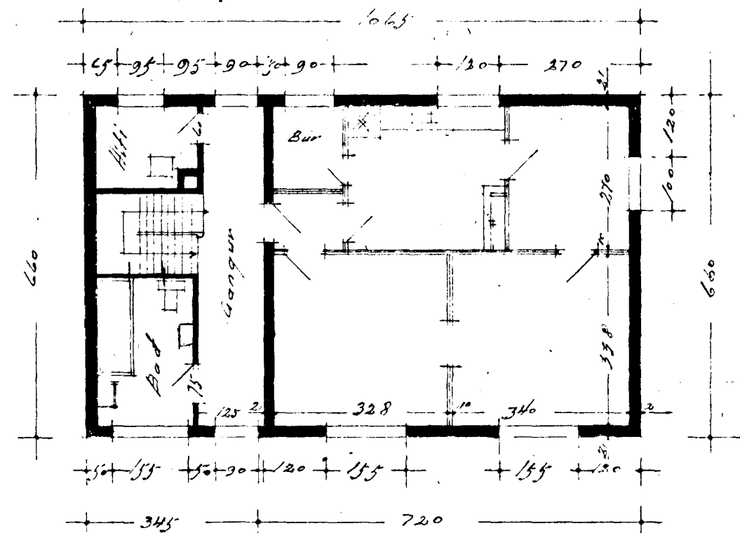
Grunnmynd
