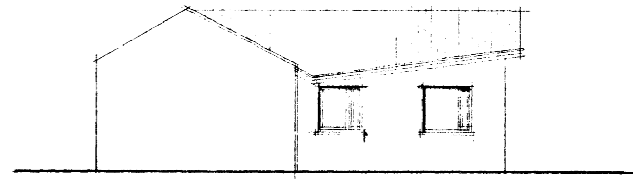
SUÐUR M=1:100
