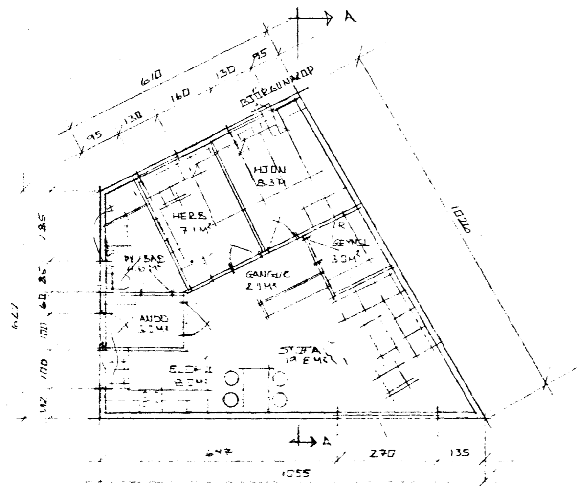
GRUNNVAND M=1:100
