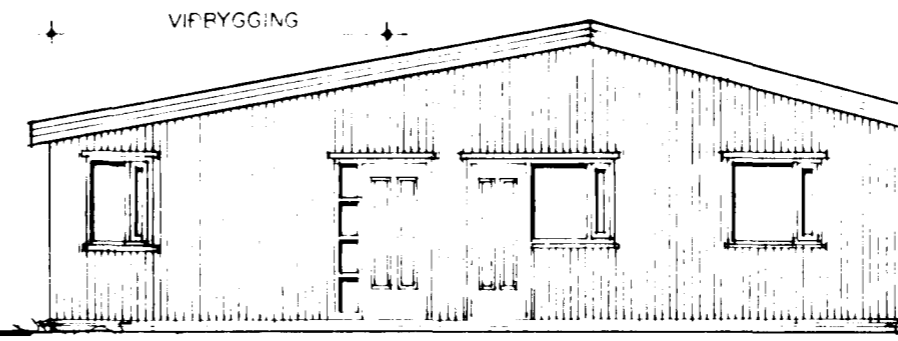
ÚTLIT SUDAUSTUR MKV. 1:100.
