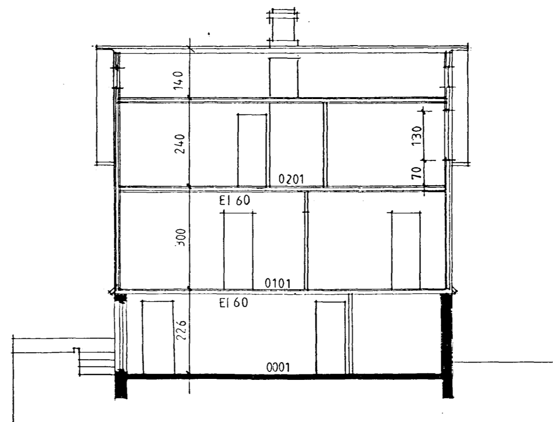
SNEIDING B - B
