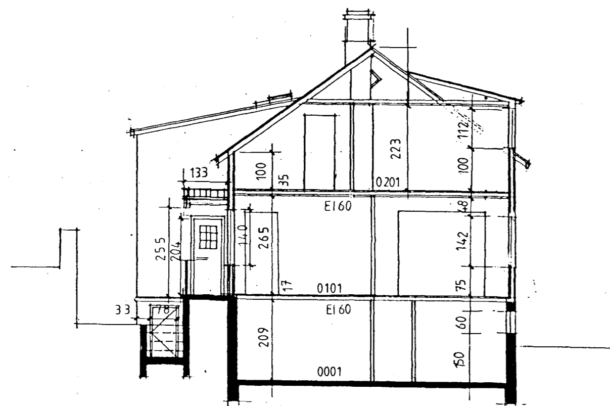
SNEIDING A - A
