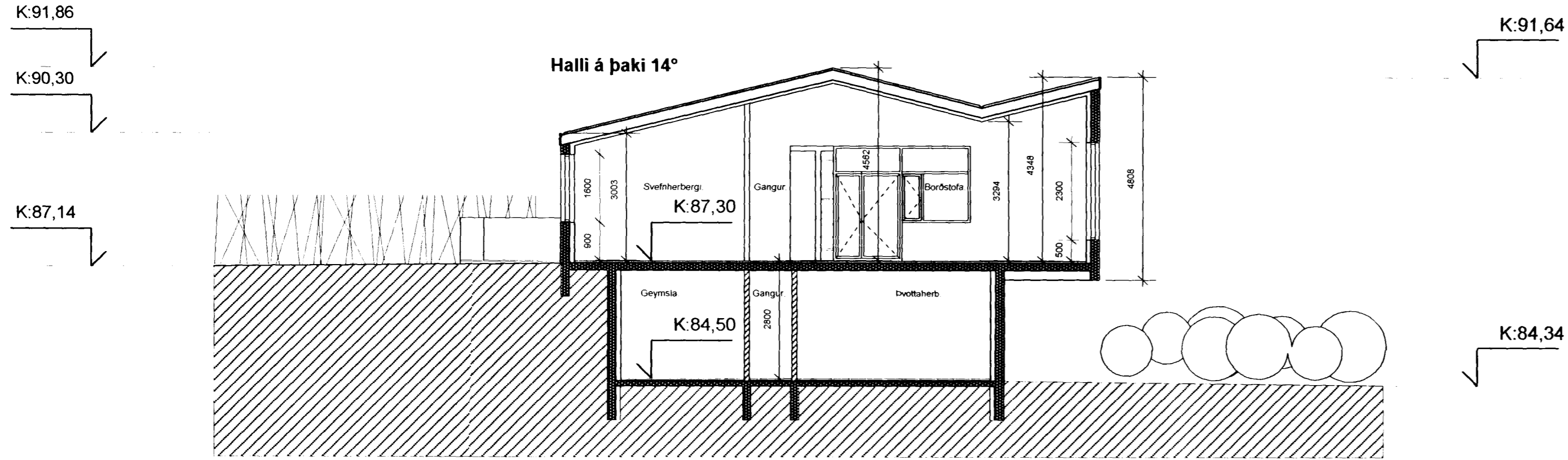
SNEIÐING A
