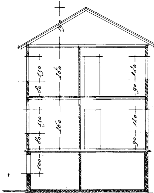
Þverska
