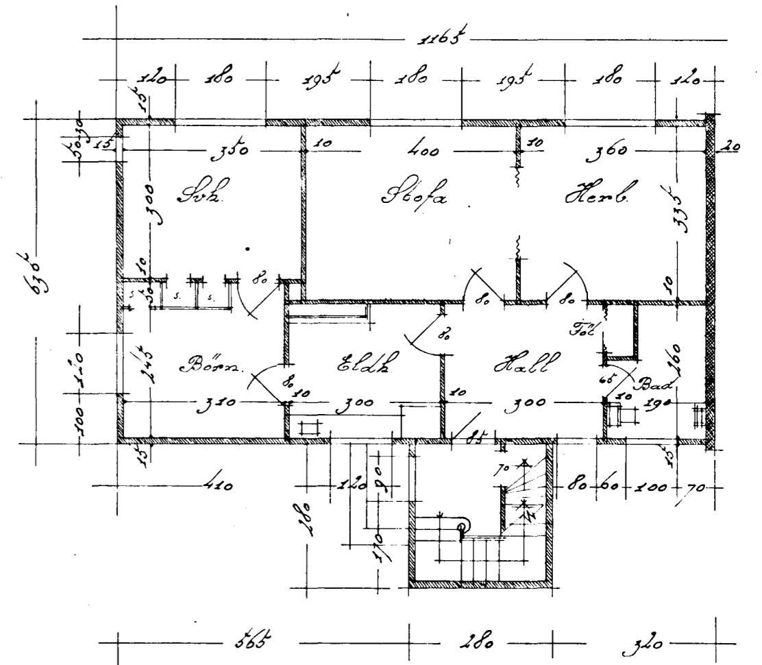
Neðri hæð
