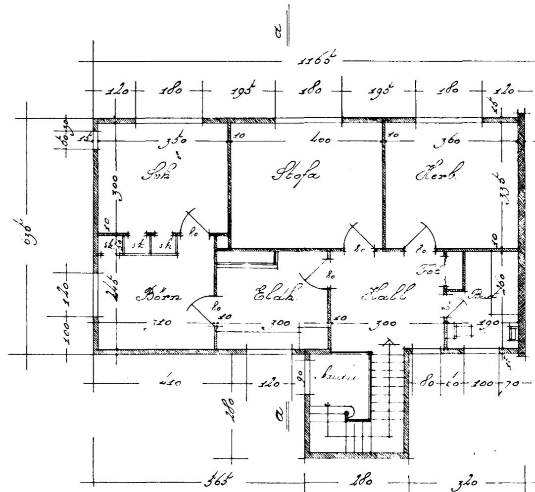
Öfri hæð
