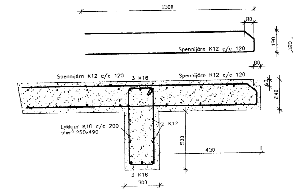
Snið B
