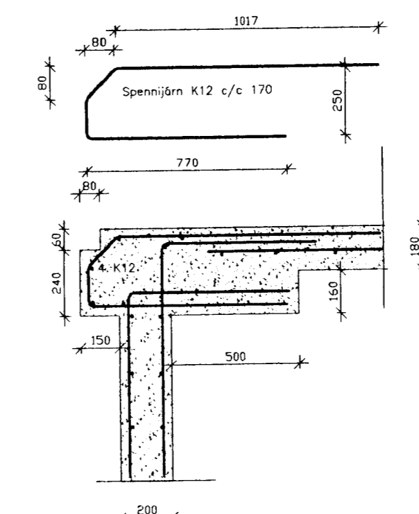
Snið A
