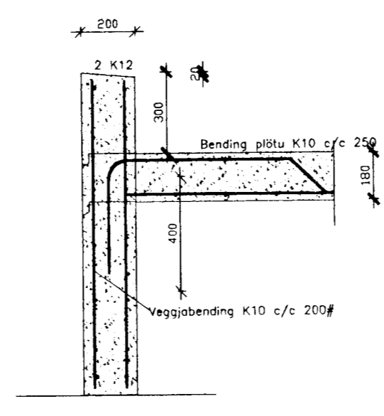
Snið C
