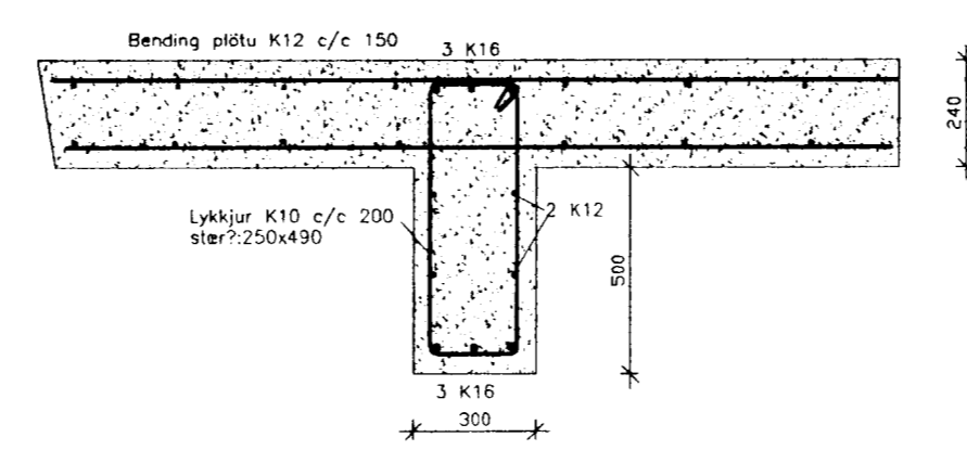
Snið D
