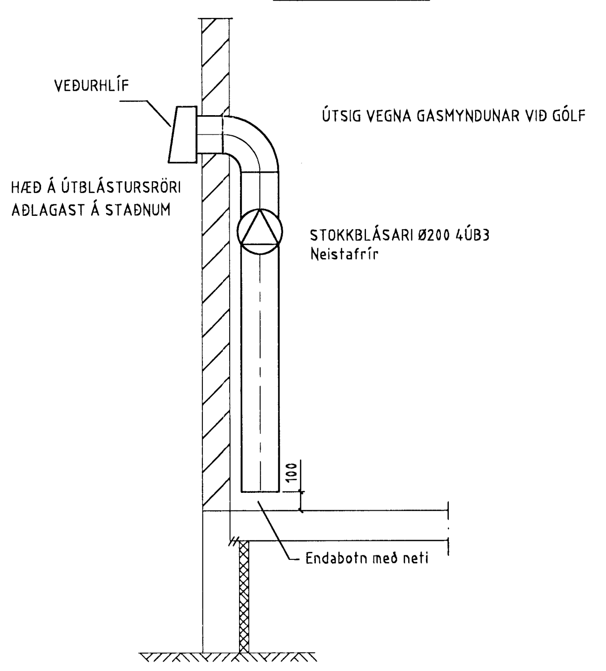
KERFI 4 ÚTSOG, MKV. 1:20
