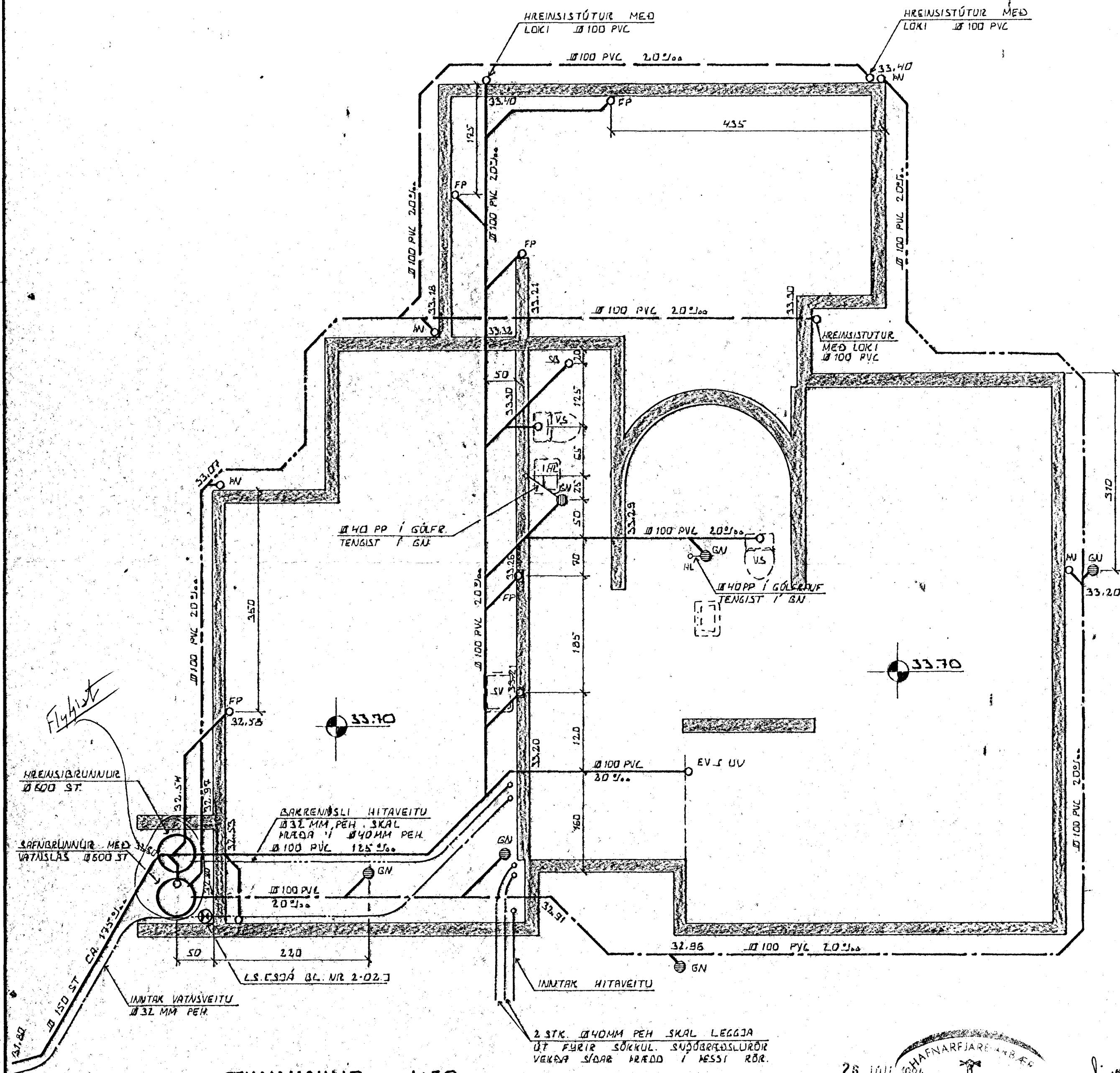
GRUNNMYND ~ 1:50
