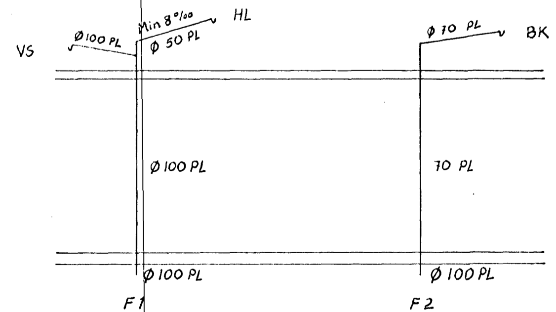
Frárennsli, fallpipur 1:50
