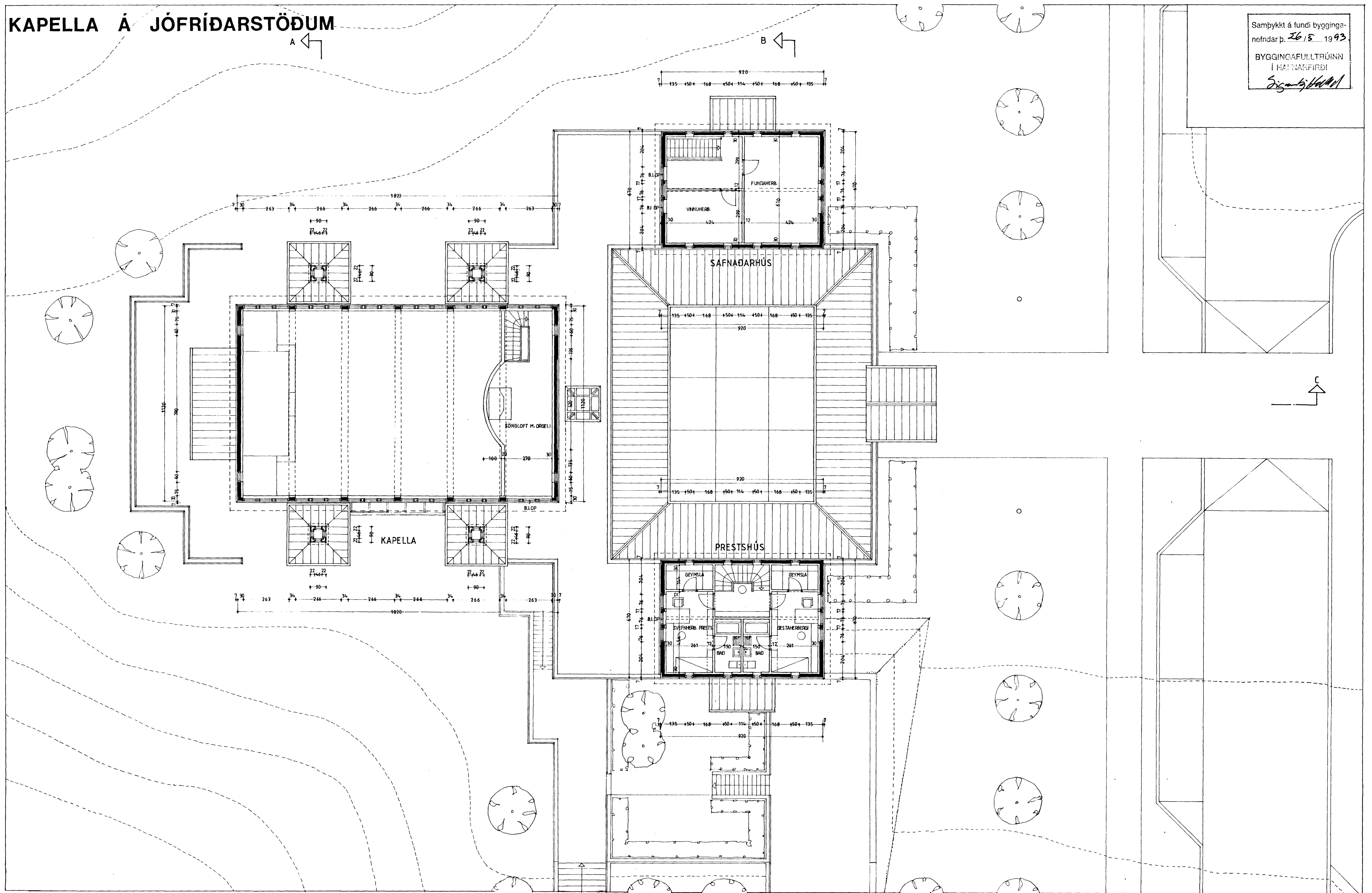
GRUNNMYND EFRÍ HÆÐAR 1:100
