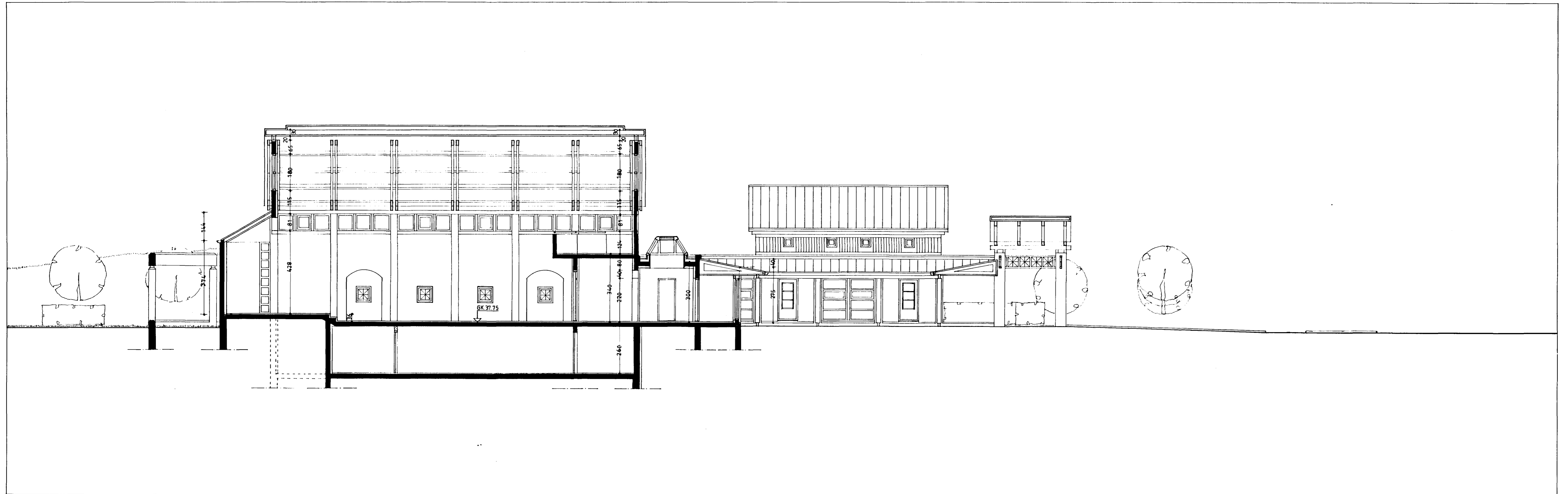
SNEIÐING C-C 1:100
