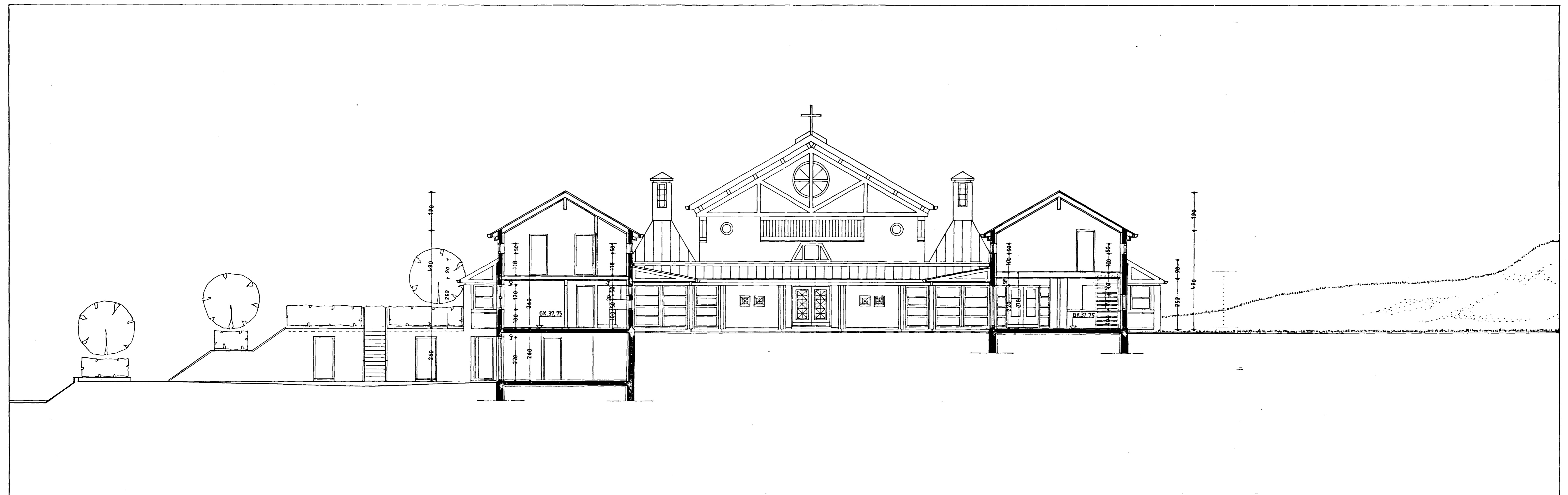
SNEIÐING B-B 1:100
