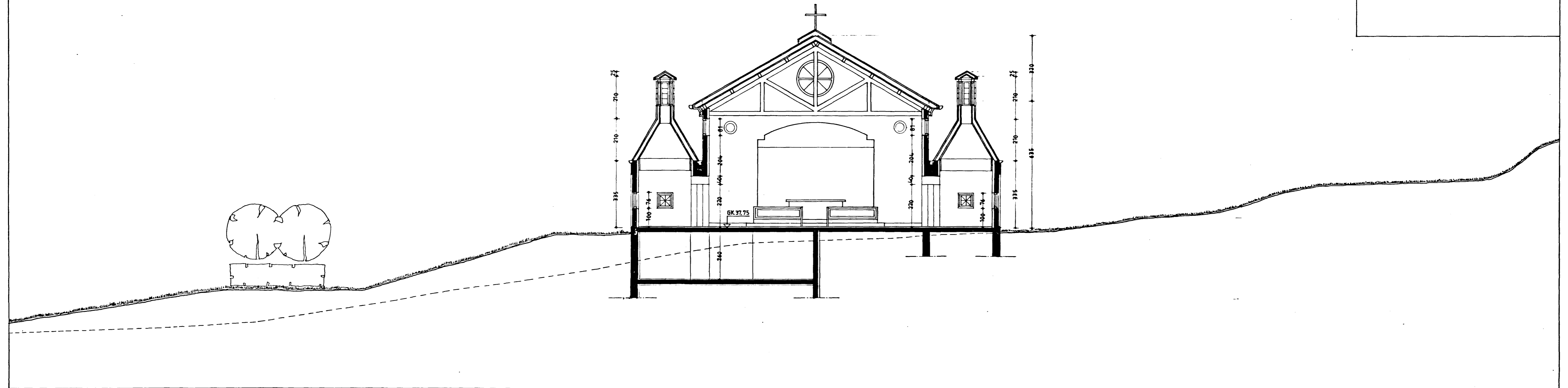
SNEIÐING A-A 1:100
