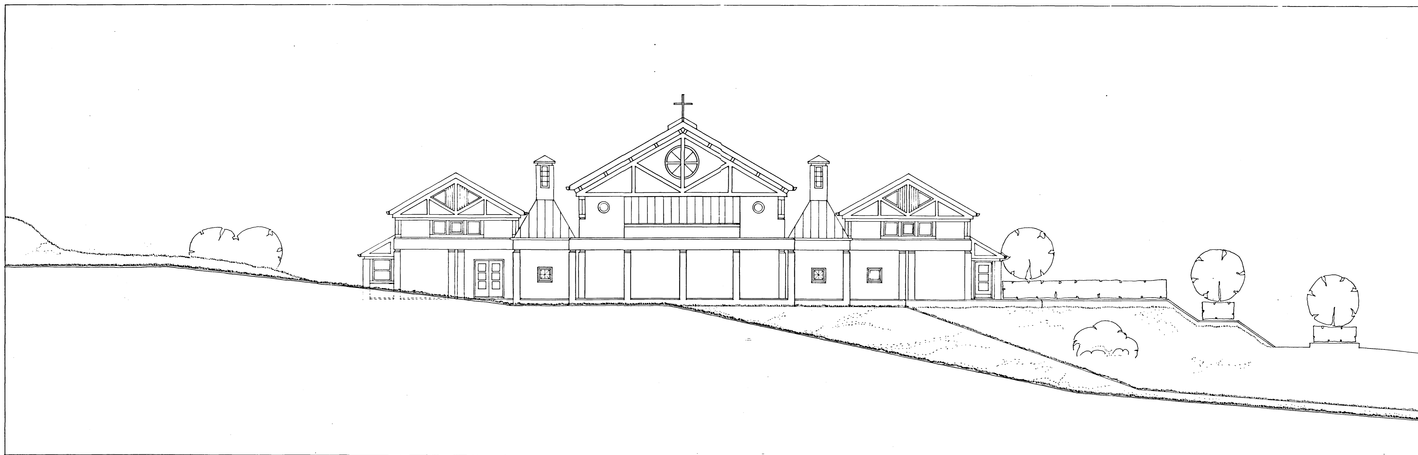
ÚTLIT TIL VESTURS 1:100
