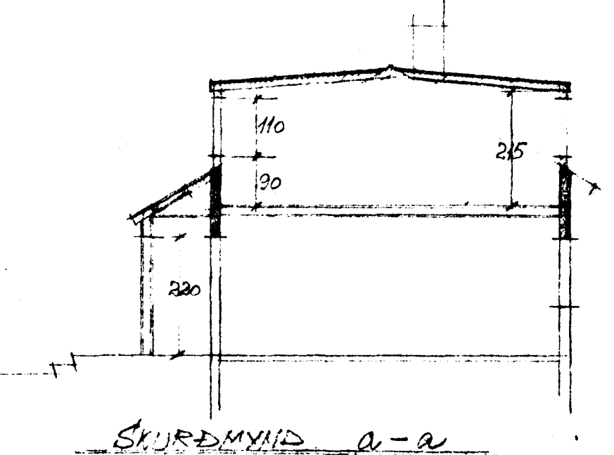
KALDAKINN 13. BREYTING A ÞAKI.
