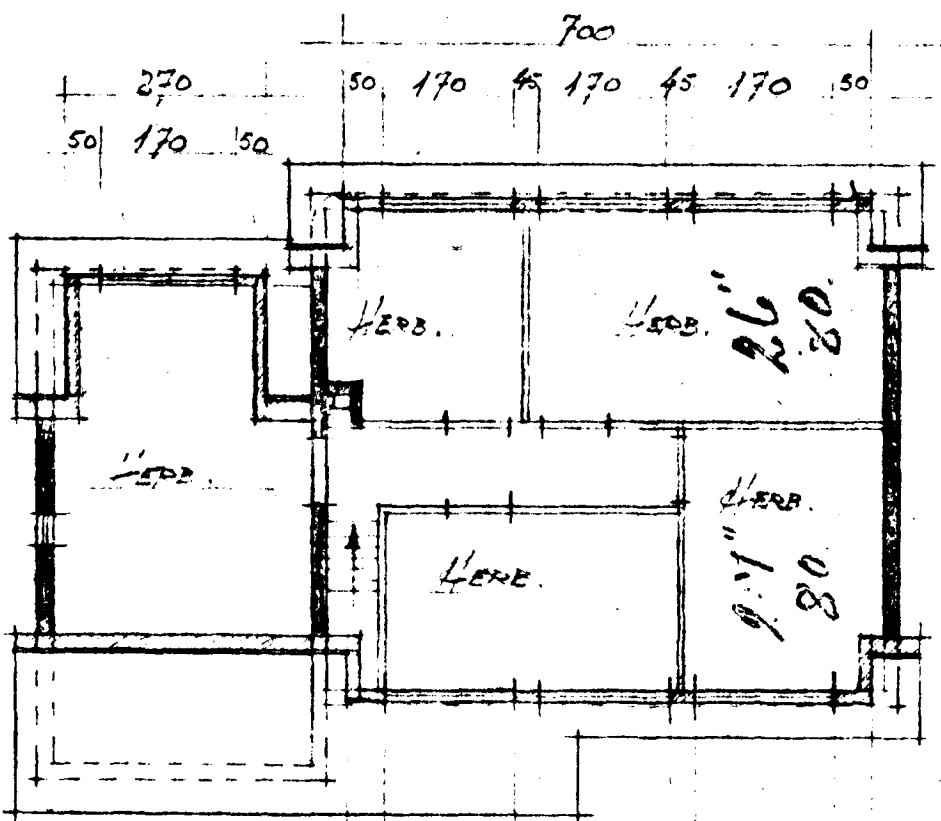
GRUNNMYND ÞAKLED
