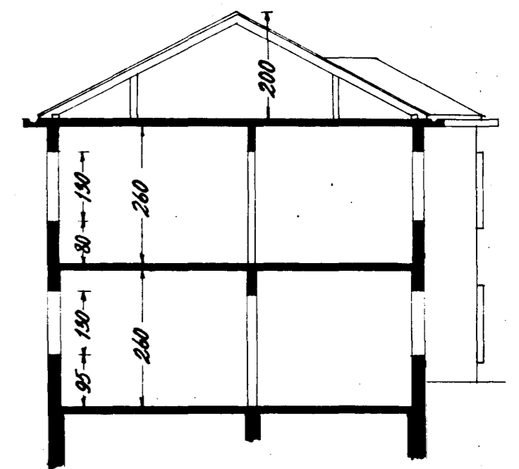
Þverskurður
