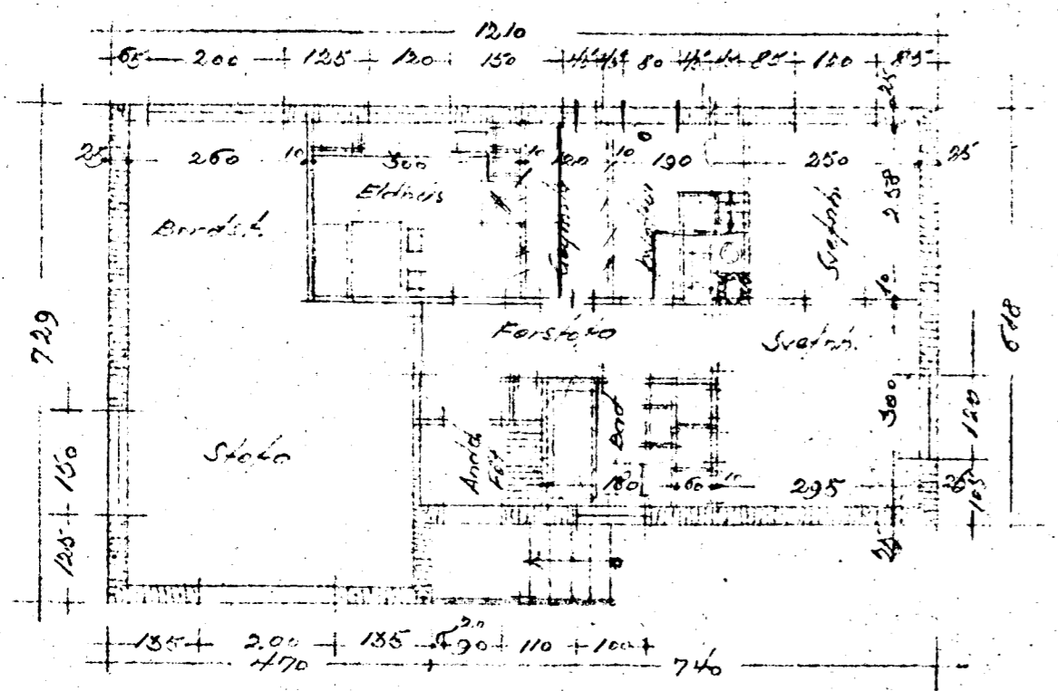
Grunnmynd
