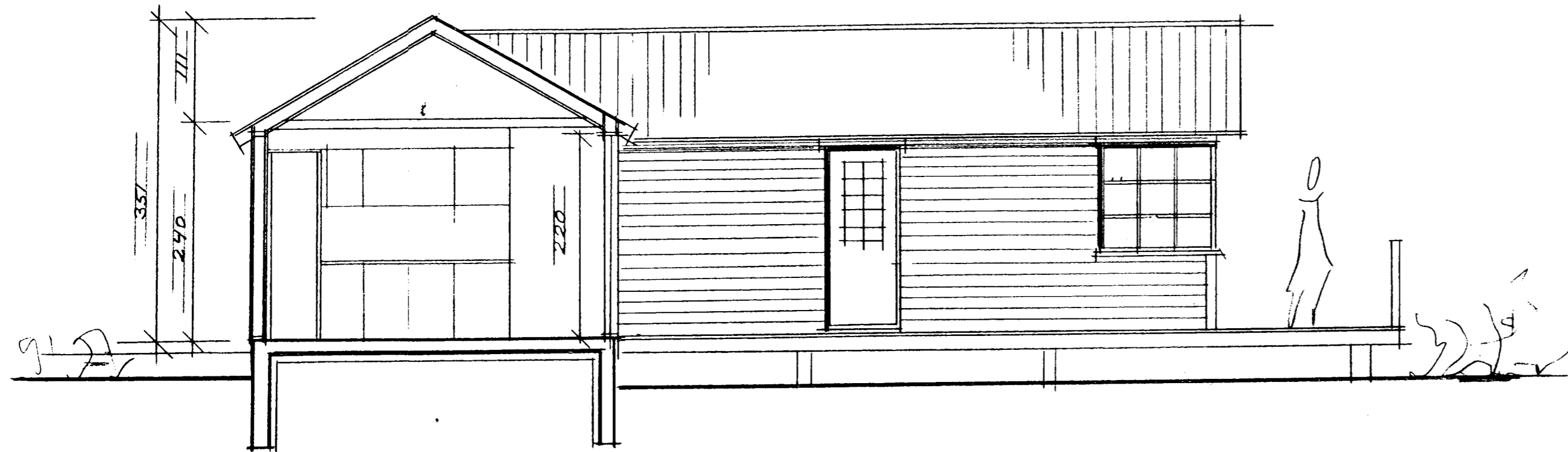
SNÍÐ A-A / ÚTLIT VESTUR M 1:50
