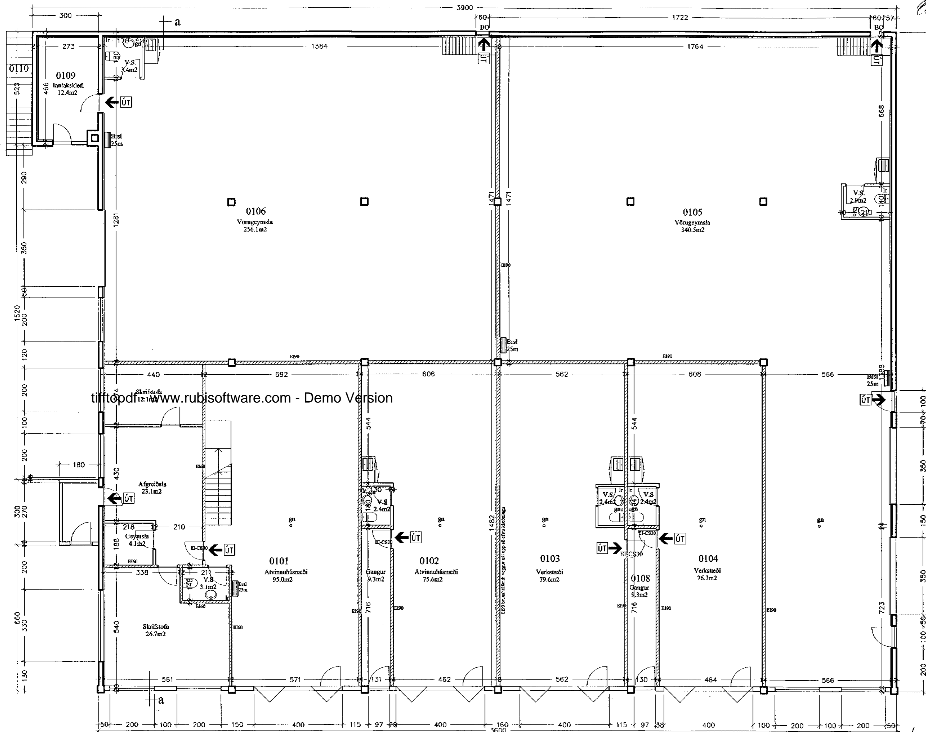
GRUNNMYND 1.HÆÐ 1:100
