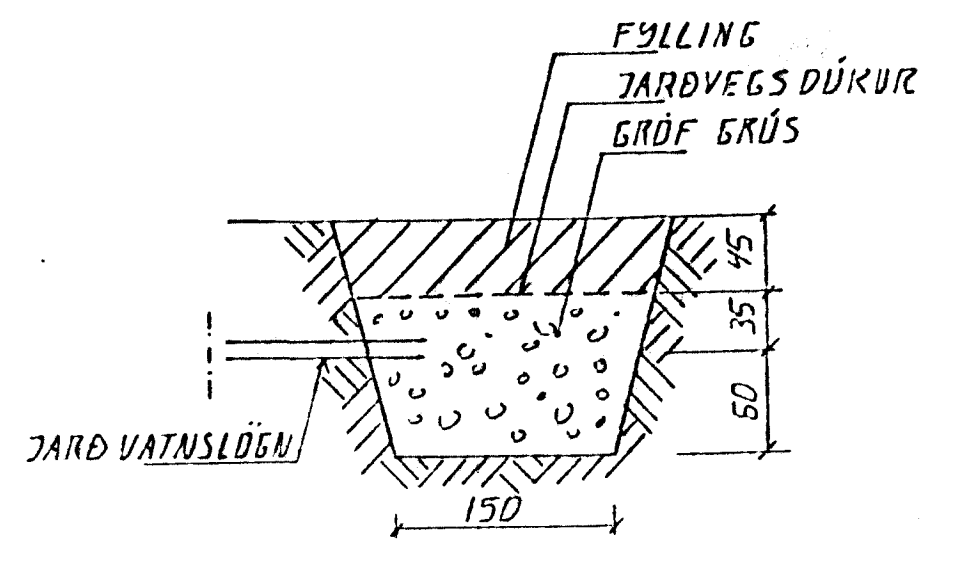
TYPISKUR GRÖÐSVELGUR 1:20
