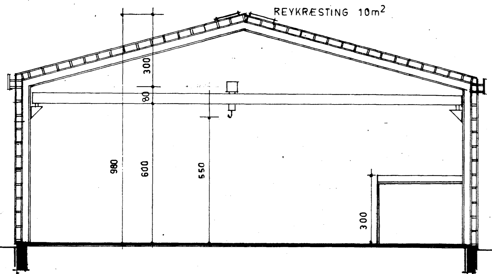
SNIÐ A — A
