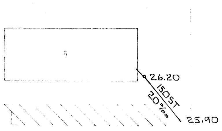
AFSTÖÐUMYND 1:500
