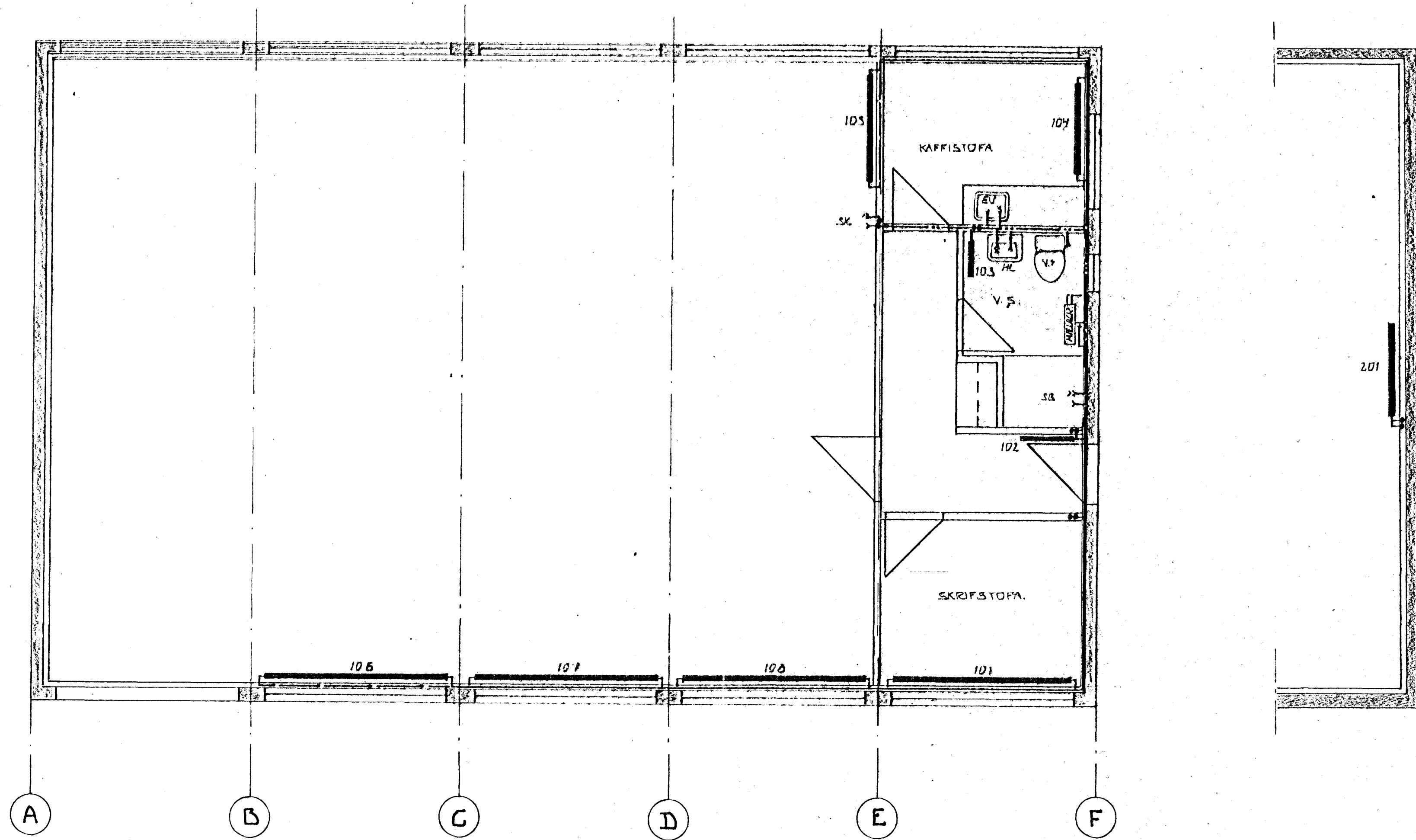
GRUNNMÝND ~ 1:50.
