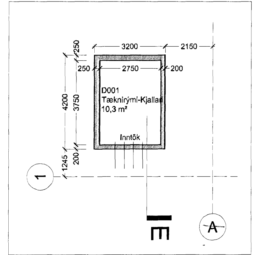
GRUNNMYND LAGNAKJALLARA í mkv. 1:100
