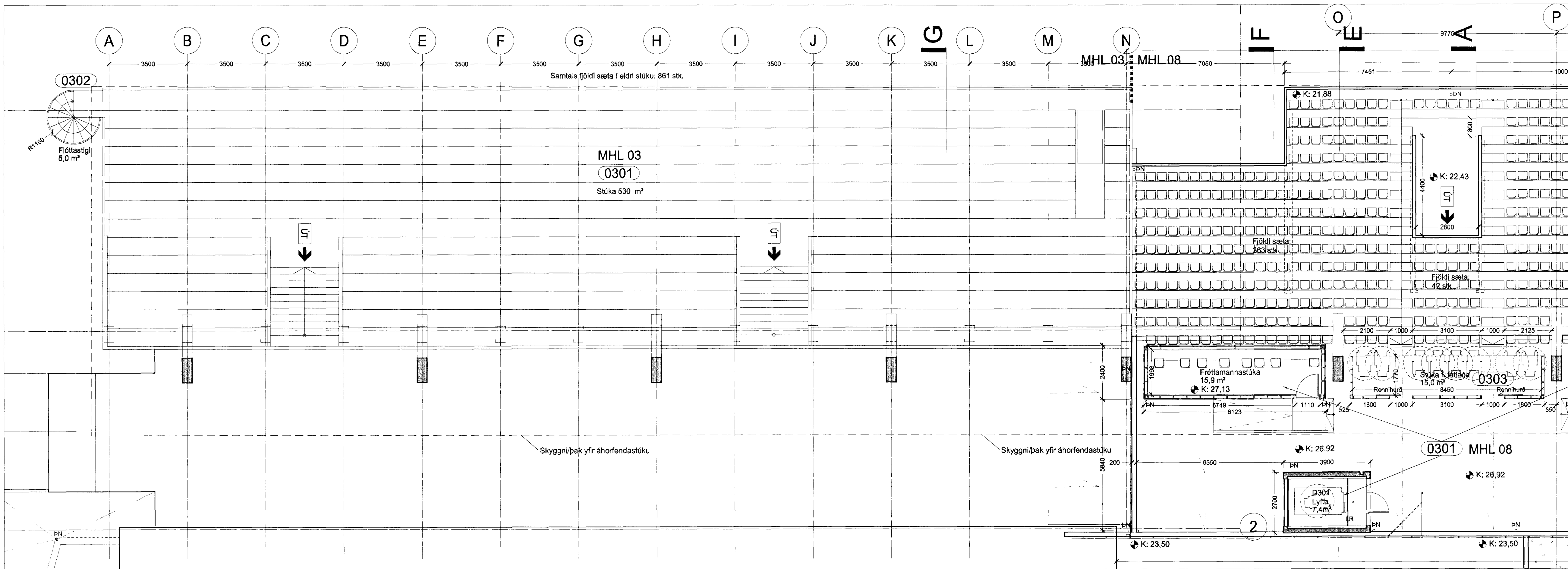
GRUNNMYND 3.HÆÐAR - SVÆÐI A í mkv. 1:100
