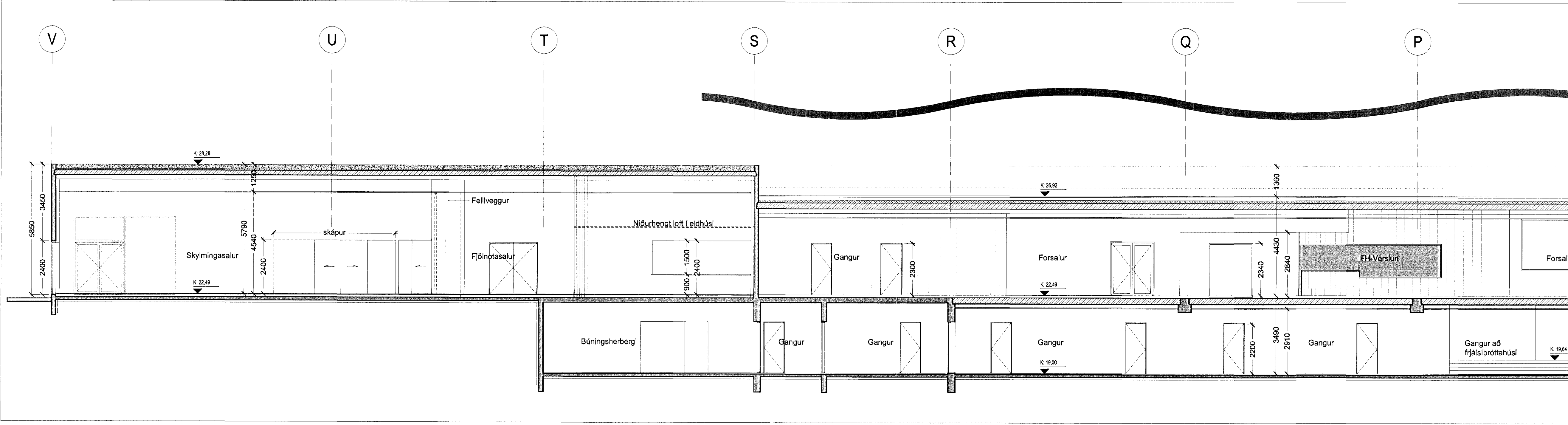
SNID B-B í mkv. 1:100
