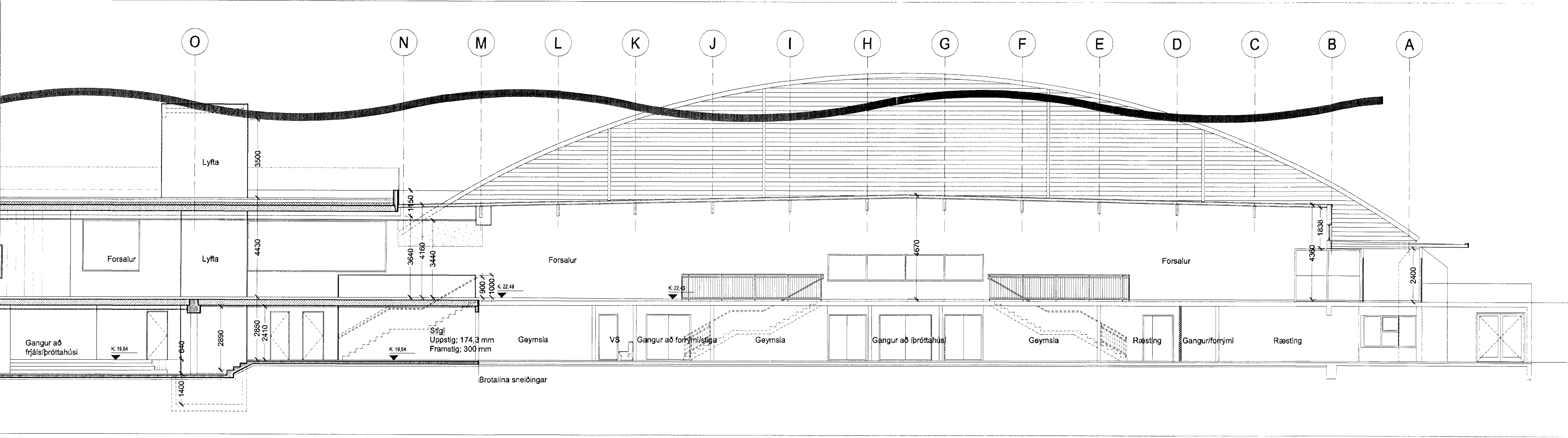
SNID B-B í mkv. 1:100
