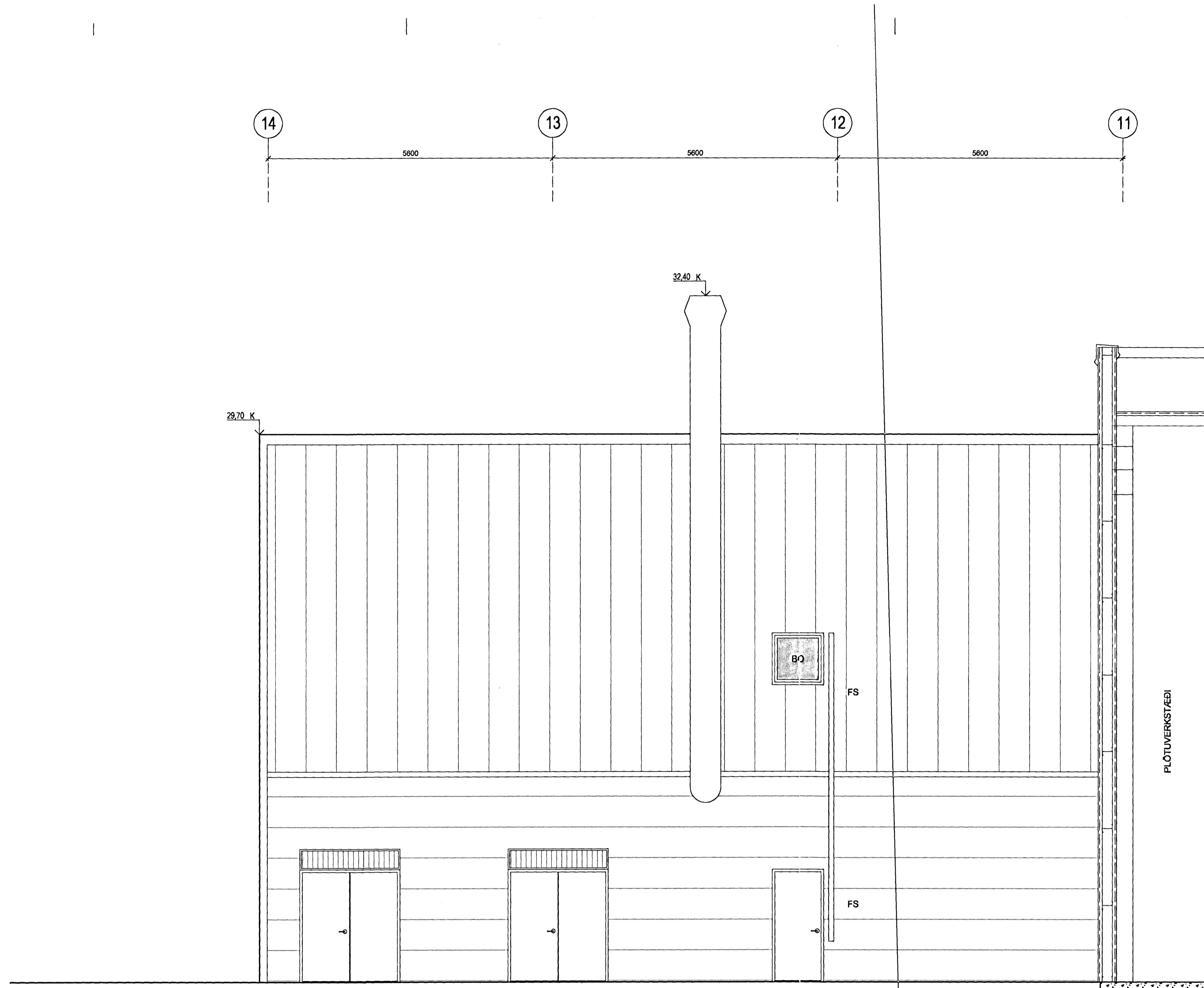
1 ÚTLIT 1:50 ÚTLIT AUSTUR (hluti)
