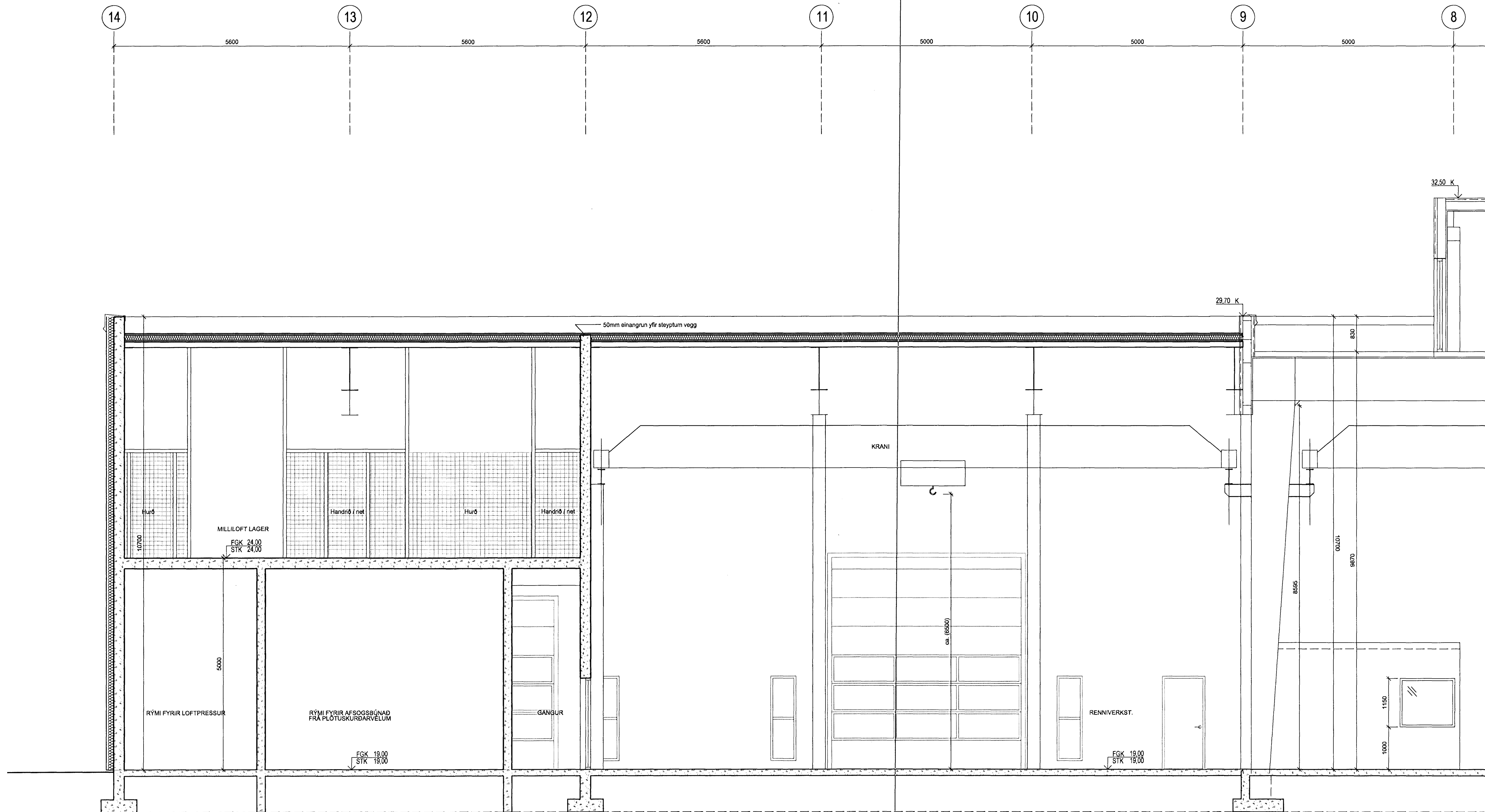
1 20-104 SNEIÐING 1:50 RENNIVERKST, TÆKINRÝMI, LAGER 20-109
