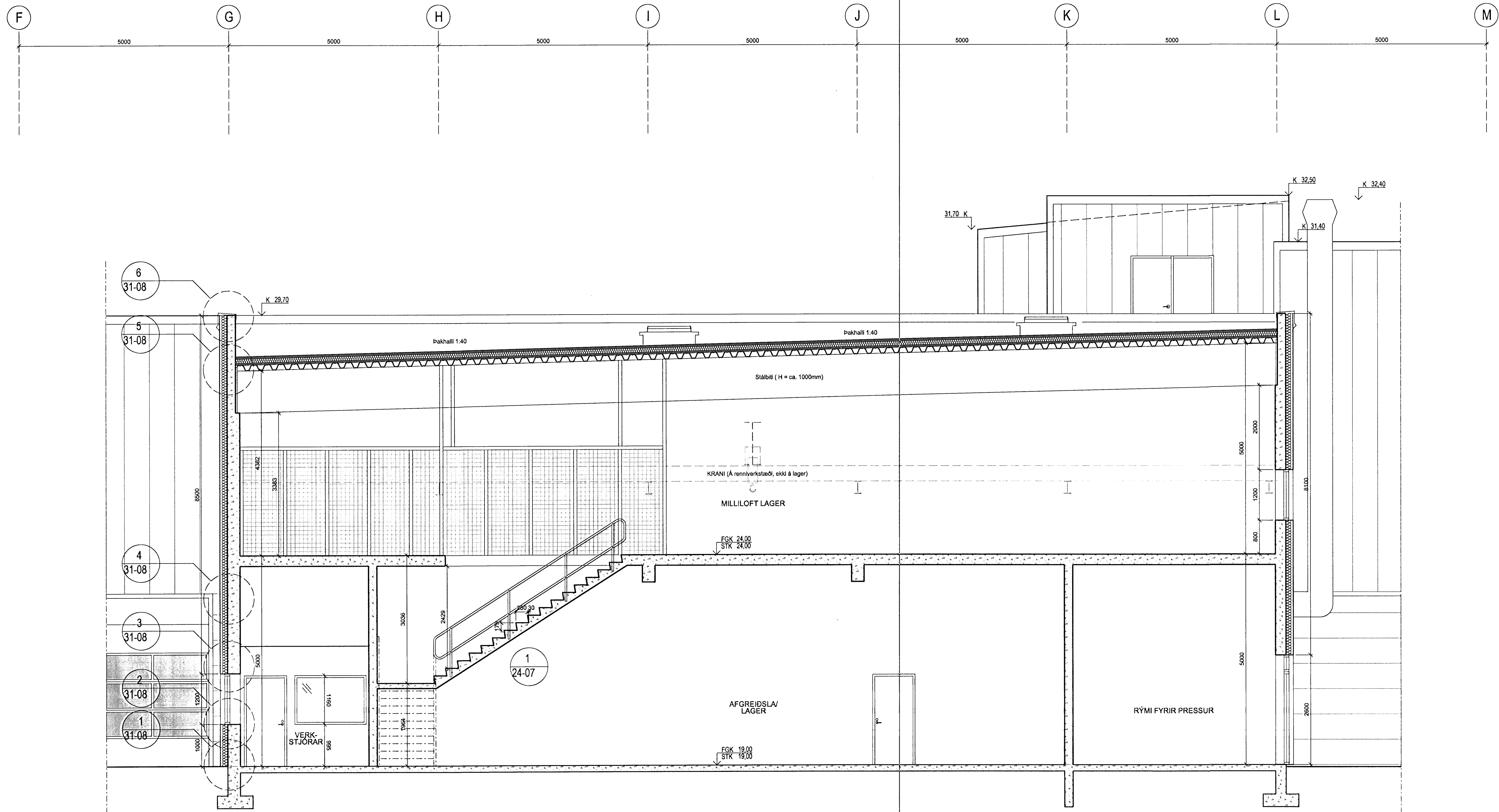
1 20-107 SNEIÐING 1:50 LAGER OG MILLILOFT YFIR LAGER
