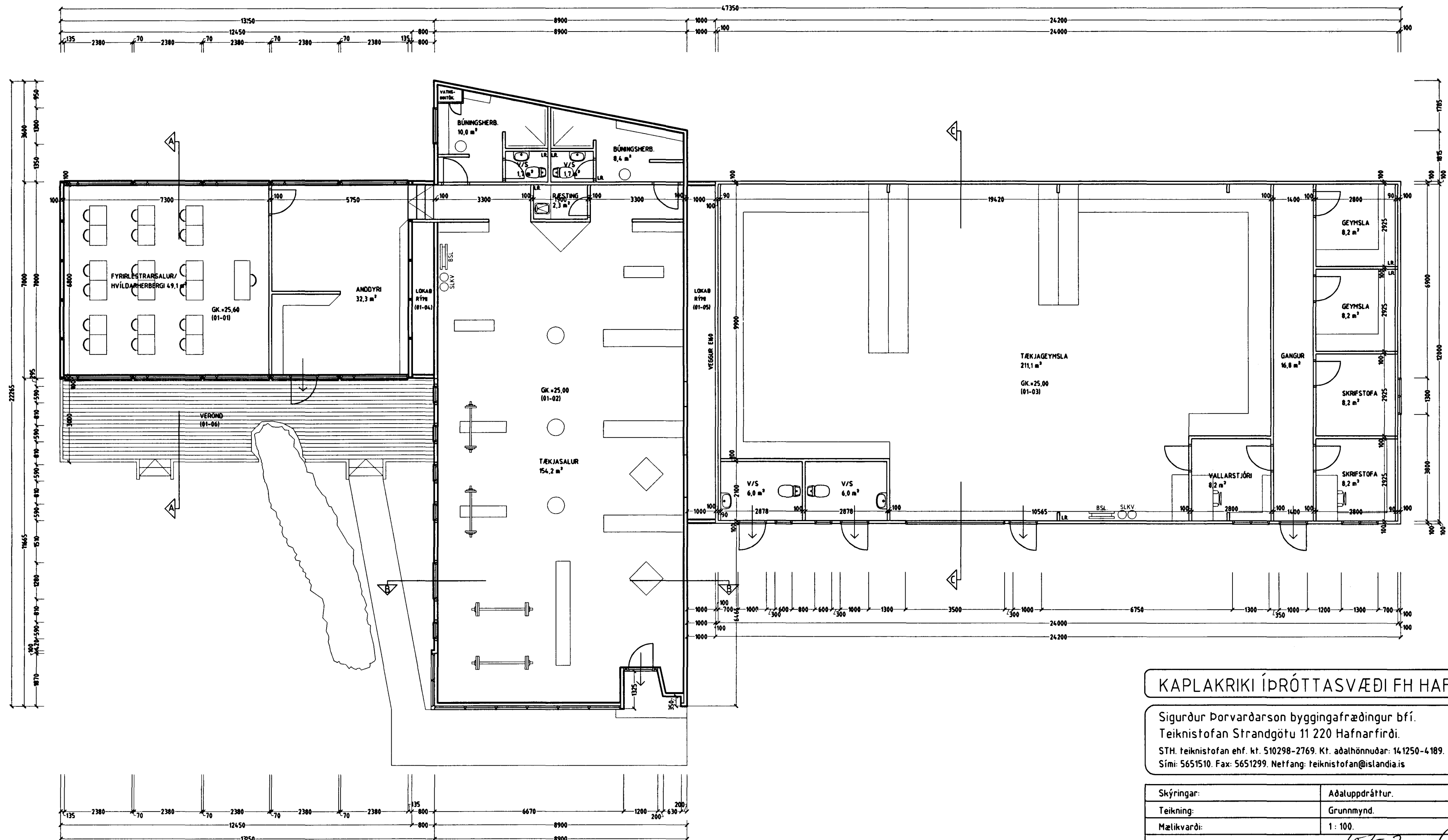
GRUNNMYND 1 HÆÐ MKV. 1:100.
