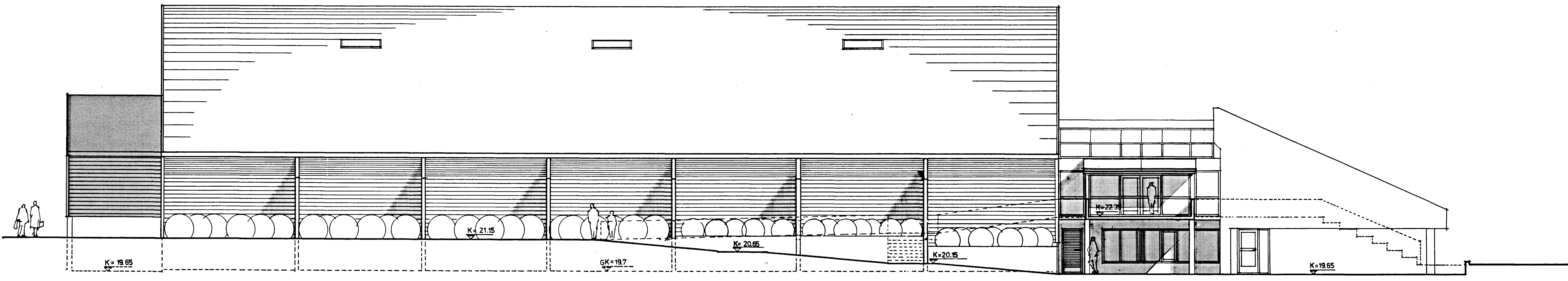
ÚTLIT Í AUSTUR mkv 1:100
