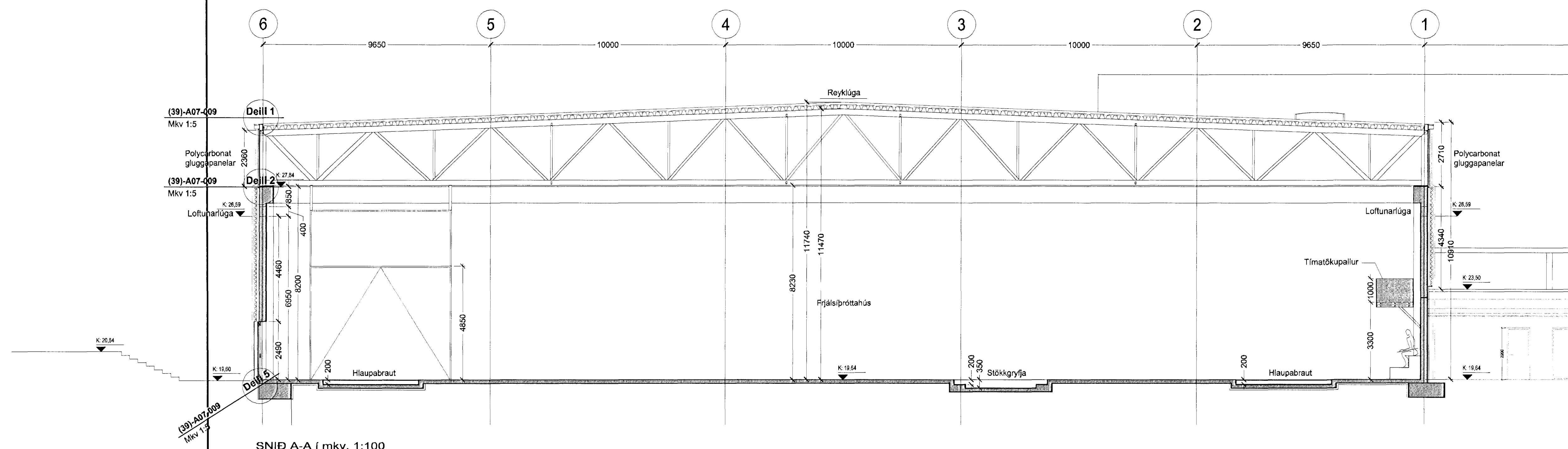
SNID A-A í mkv. 1:100
