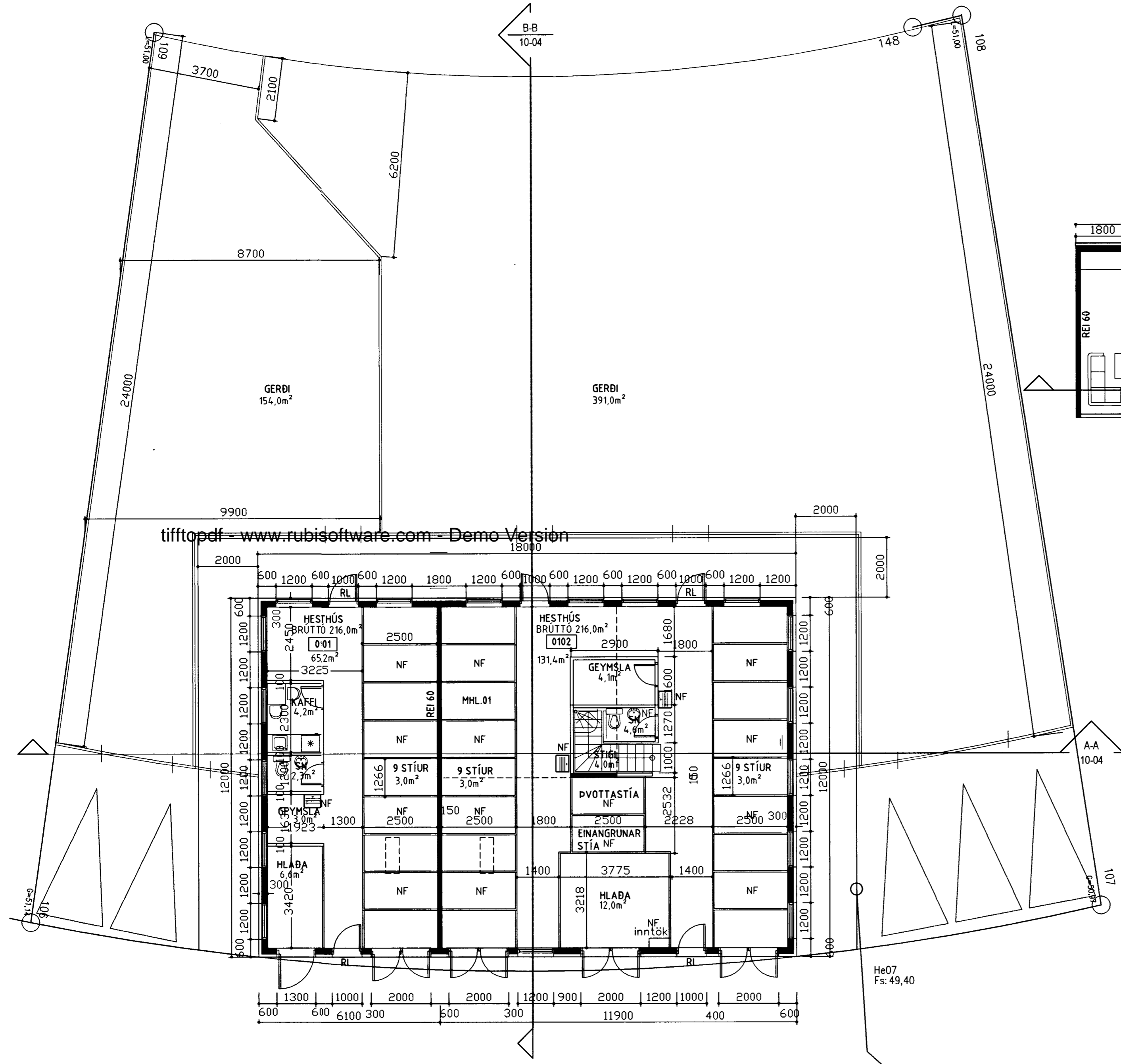
GRUNNMYND 1.HÆÐ 1:100
