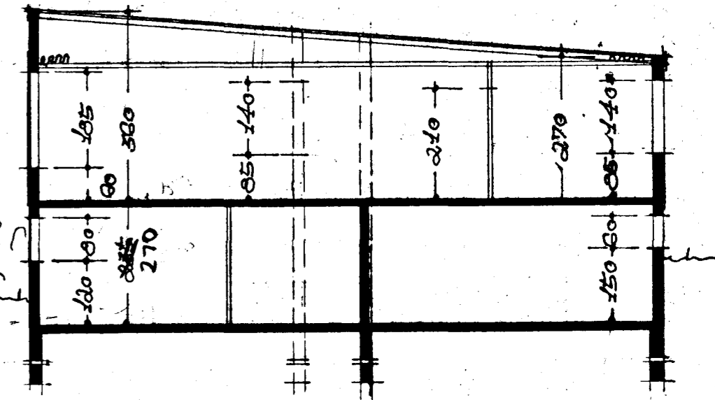
SKURÐUR A-A
