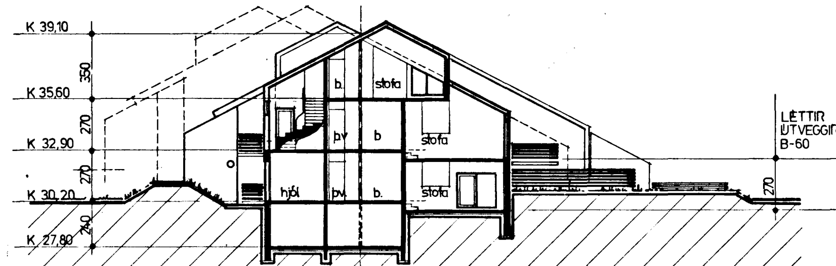
sneiding b-b
