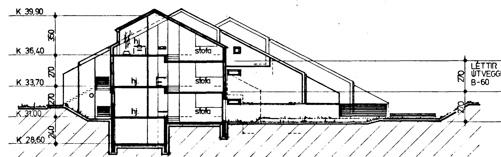
sneiding c-c
