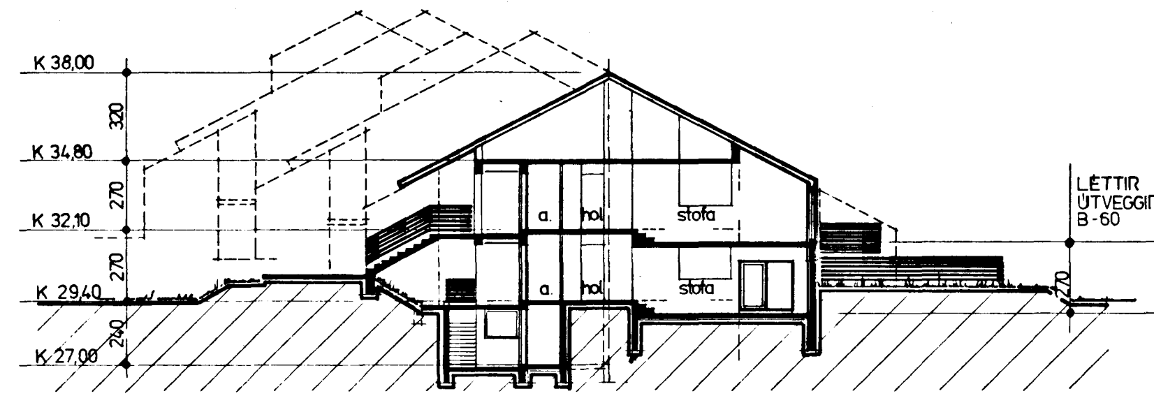
sneiding a-a
